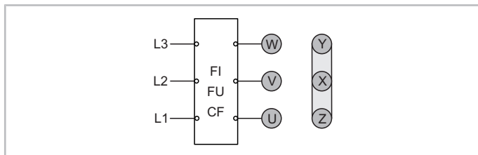
Рис. 14: Клеммы мотора на клеммной плите для работы с внешним преобразователем частоты (FI) для поршневых компрессоров с мотором 40S и подключением звездой
