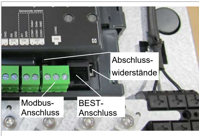
Abb. 11: Modbus-/BEST-Anschluss am CSV. Verdichter
