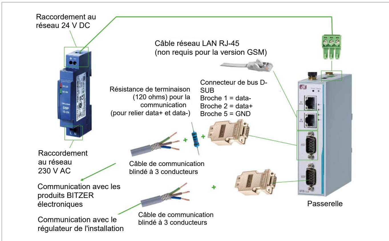
Fig. 26: Raccordement de la passerelle dans une configuration en pont
