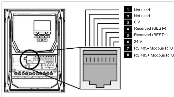
Fig. 14: Raccorder le convertisseur de fréquences à un PC via le convertisseur d'interface BEST et le câble adaptateur RJ45 marqué en bleu
