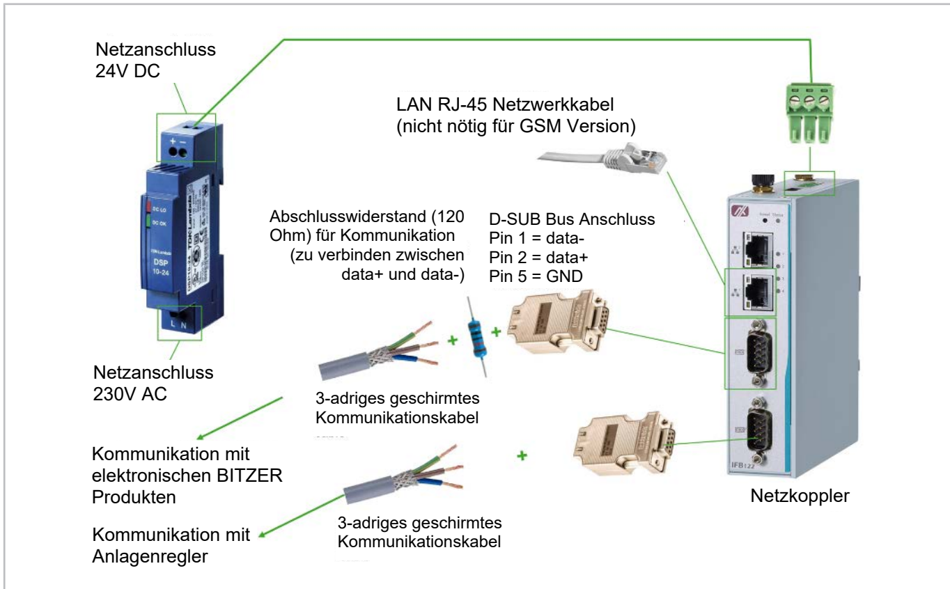
Abb. 26: Anschluss des Netzkopplers in einer Brückenkonfiguration
