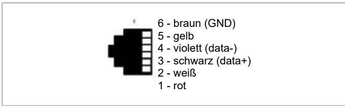
Abb. 12: RJ12-Anschluss der Pins für den BEST-Anschluss an CSV und SE-i1
