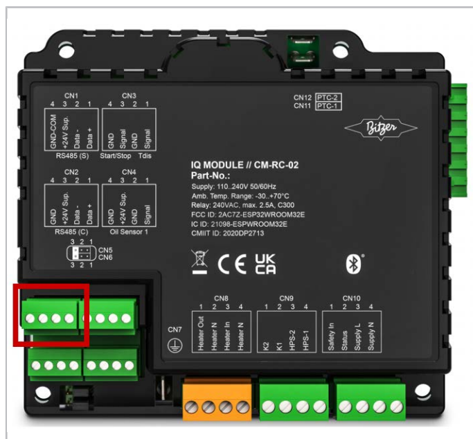
Fig. 8: Connecteur Modbus pour la communication avec la passerelle sur IQ MODULE CM-RC-02
