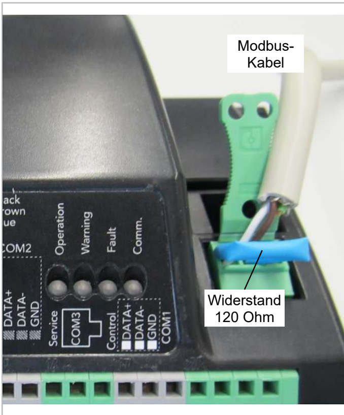
Abb. 10: Modbus-Anschluss am SE-i1
