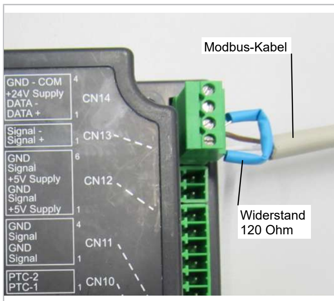
Abb. 9: Modbus- /BEST-Anschluss am CM-SW-01 oder CM-RC-01 (beide Protokolle sind am gleichen Anschluss möglich)
