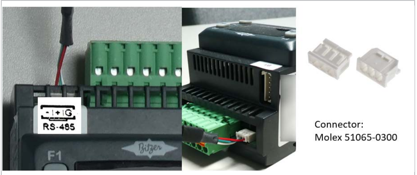
Abb. 16: Modbus-Anschluss am ECOLITE Regler
