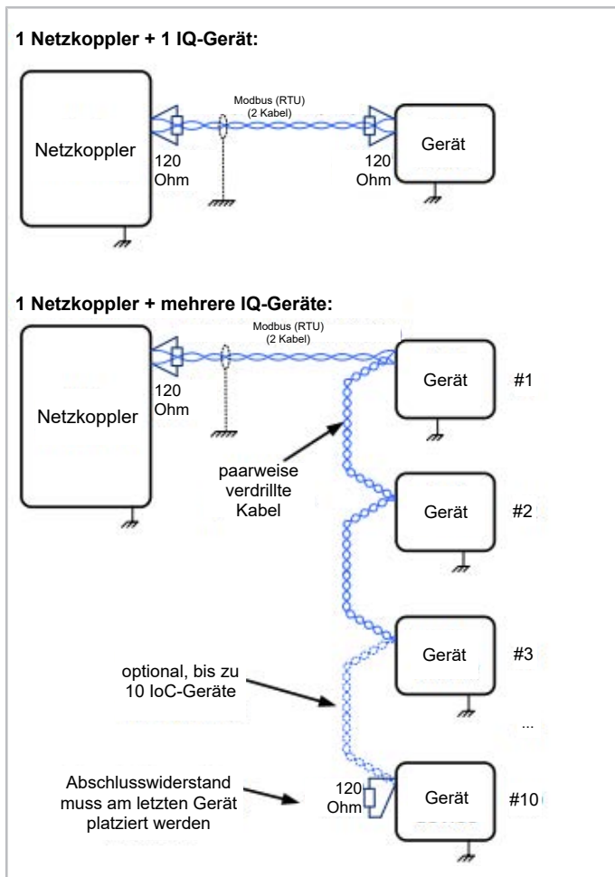
Abb. 5: Korrekte Modbus-Schaltung
