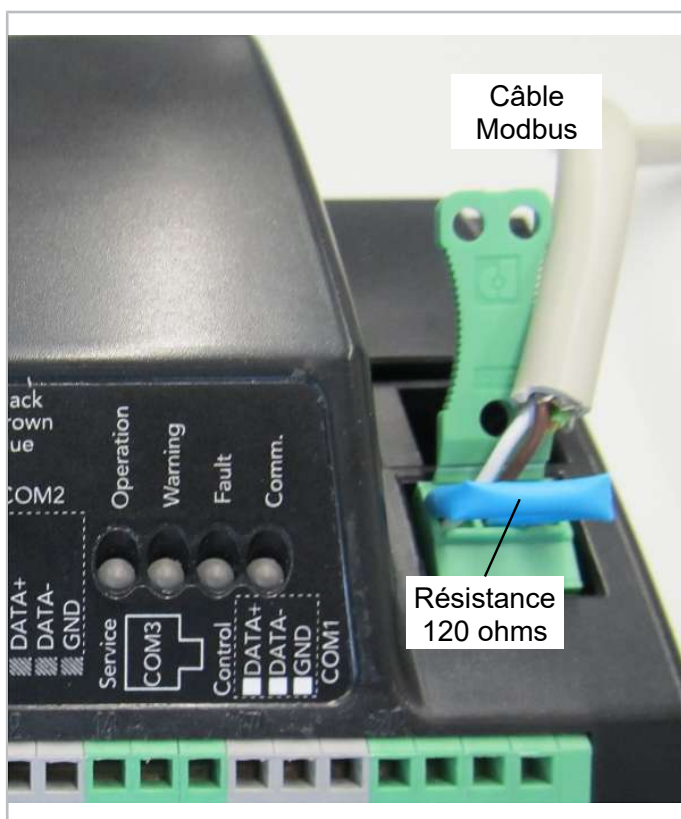
Fig. 10: Raccord Modbus sur SE-i1
