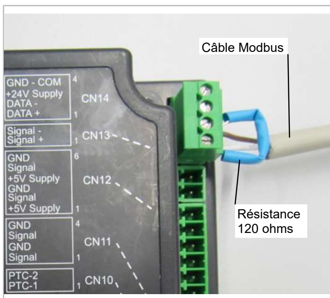
Fig. 9: Raccord Modbus/BEST sur CM-SW-01 ou CM-RC-01 (les deux protocoles sont possibles sur le même raccord)
