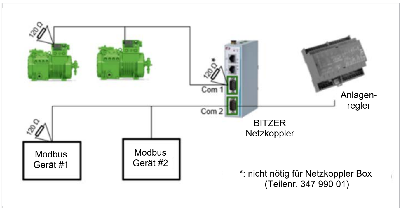
Abb. 25: Brückenkonfiguration: allgemeine Einrichtung
