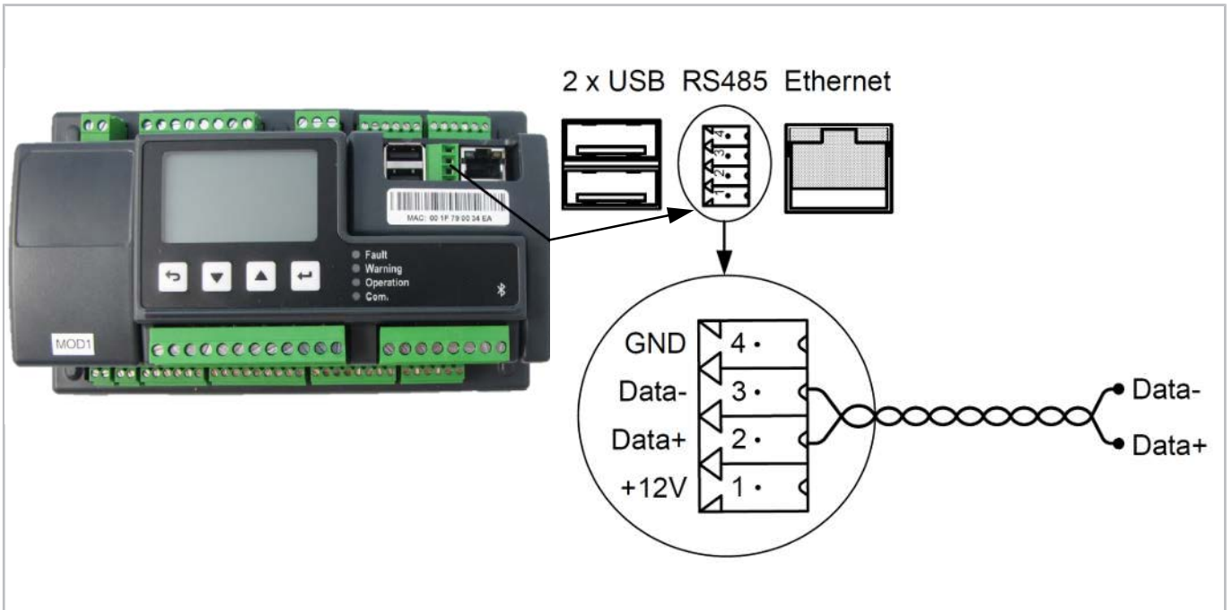
Abb. 15: Modbus-Anschluss am ECOSTAR Regler
