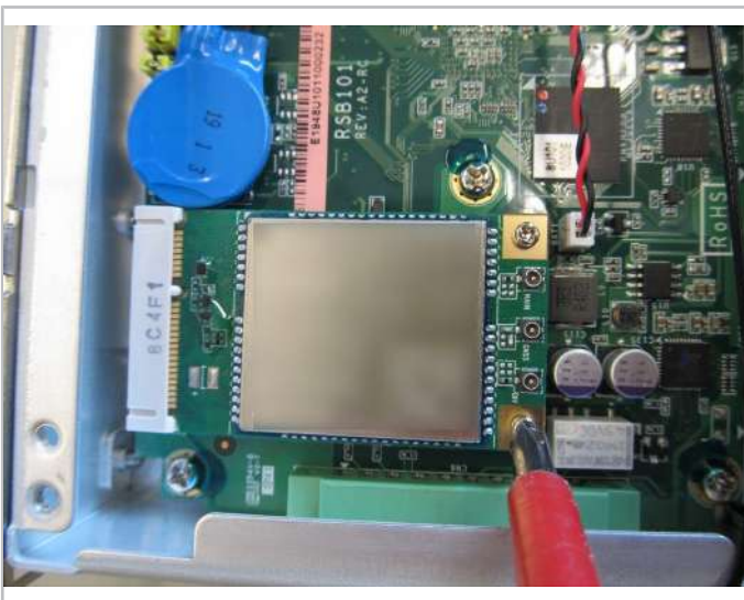
Abb. 19: Schrauben am GSM-Modul lösen.
