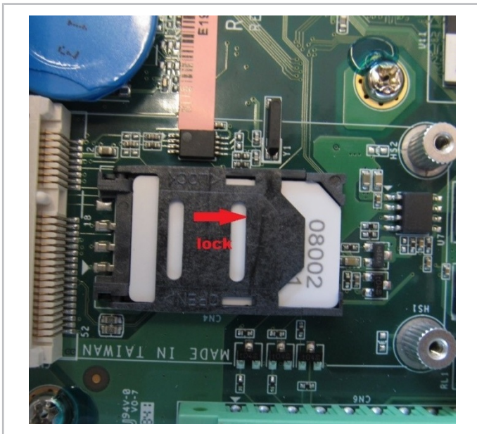
Abb. 22: SIM-Karte einstecken, Halter verriegeln.
