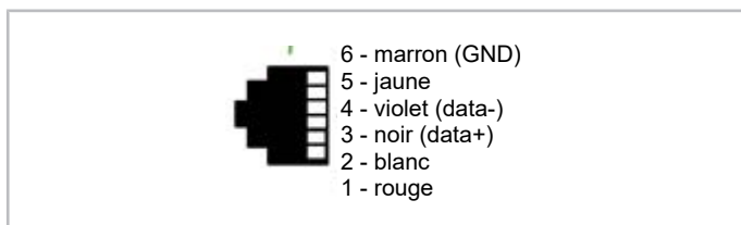
Fig. 12: Connecteur RJ12 des broches pour le raccord BEST sur CSV et SE-i1
