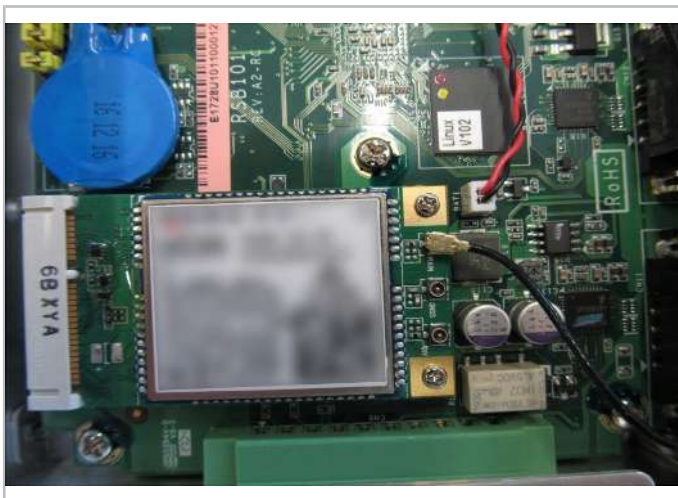
Fig. 23: Remonter le module GSM et raccorder le câble d'antenne.
