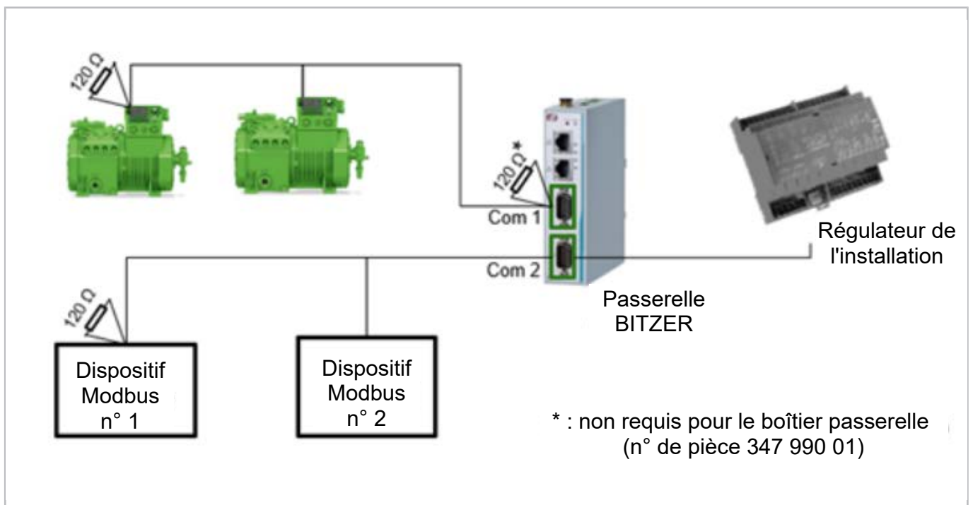
Fig. 25: Configuration en pont : paramétrage général
