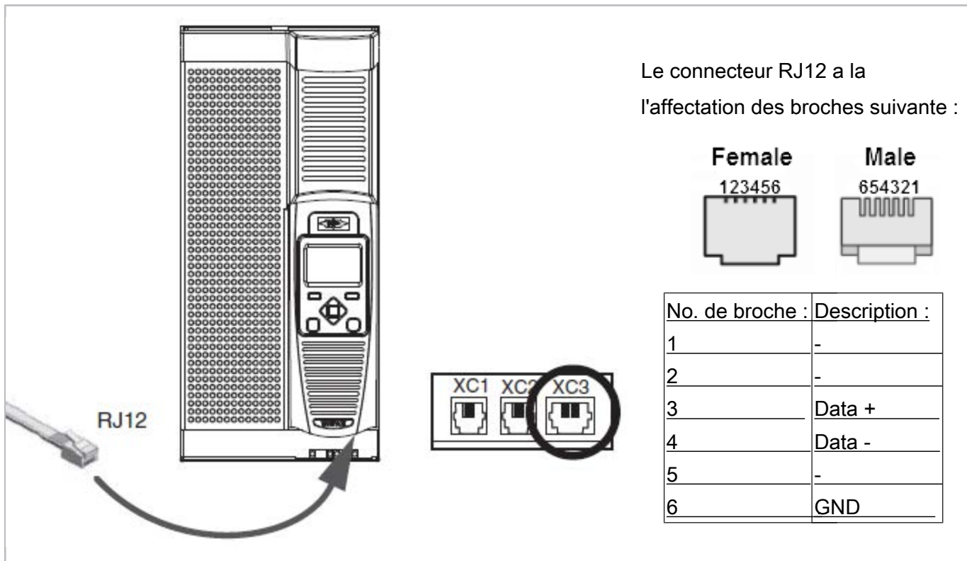
Fig. 13: Bornes de la prise d'interface Modbus du VARIPACK
