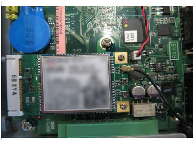
Abb. 23: GSM-Modul wieder einbauen und Antennenkabel anschließen.
