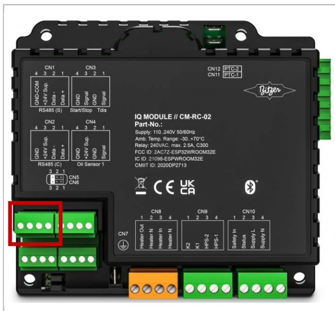
Abb. 8: Modbus-Anschluss für die Kommunikation mit dem Netzkoppler am IQ MODUL CM-RC-02
