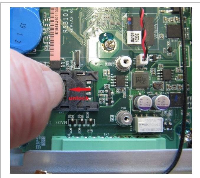
Fig. 21: Déverrouiller le support de carte SIM.
