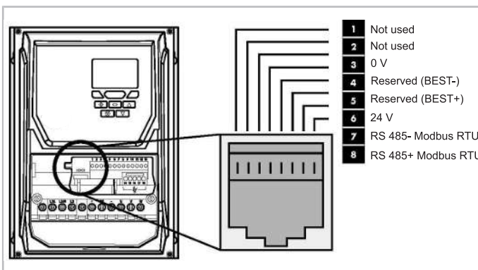
Abb. 14: Den Frequenzumrichter über den BEST Schnittstellenkonverter und das blau gekennzeichnete RJ45-Adapterkabel an einen PC anschließen
