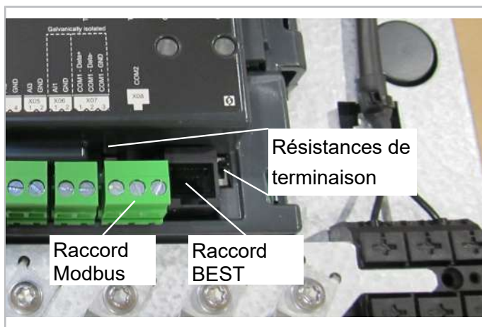
Fig. 11: Raccord Modbus/BEST sur le compresseur CSV.
