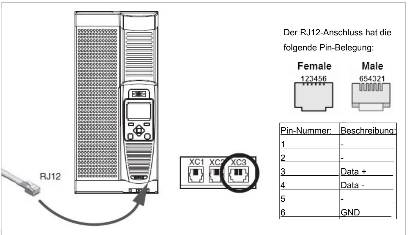
Abb. 13: Klemmen der Modbus-Schnittstellenbuchse des VARIPACK
