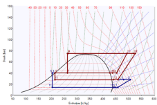
Darstellung des Prozesses im Druck-Enthalpie Diagramm
