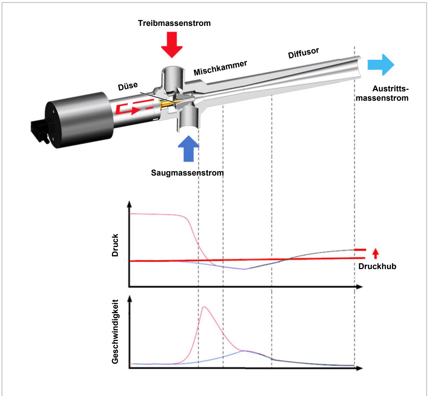
Abb. 19: Schematische Darstellung eines regelbaren Hochdruck-Ejektors mit Druck- und Geschwindigkeitsverlauf der Massenströme
