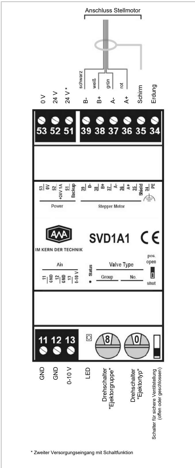
Abb. 29: Steuergerät SVD1A1
