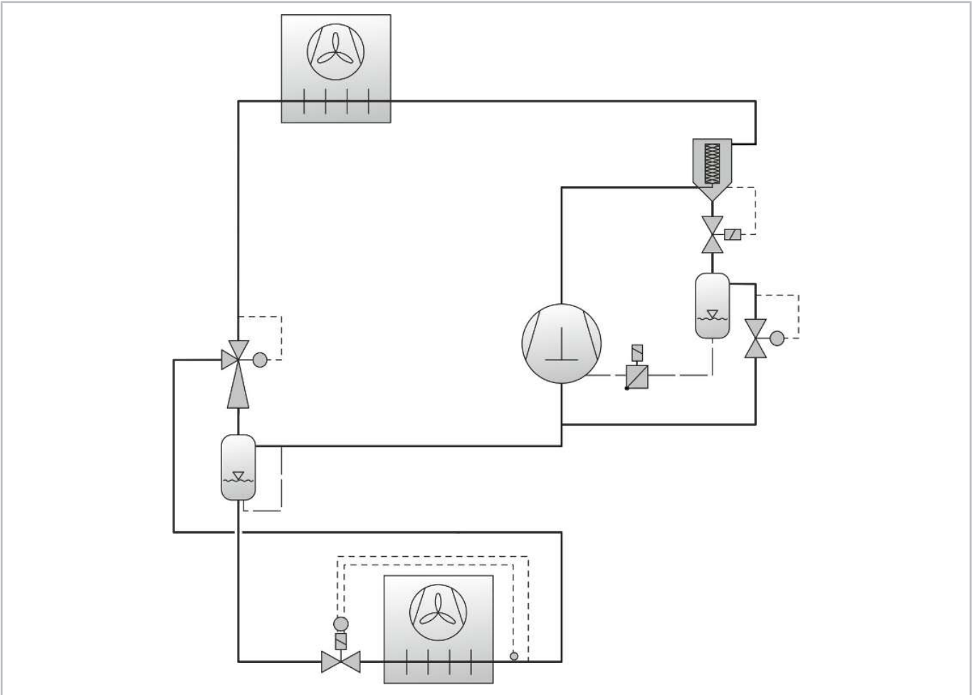
Abb. 21: Anlagenschema: Ejektor in Low-Lift-Anwendung (vereinfachte Darstellung)
