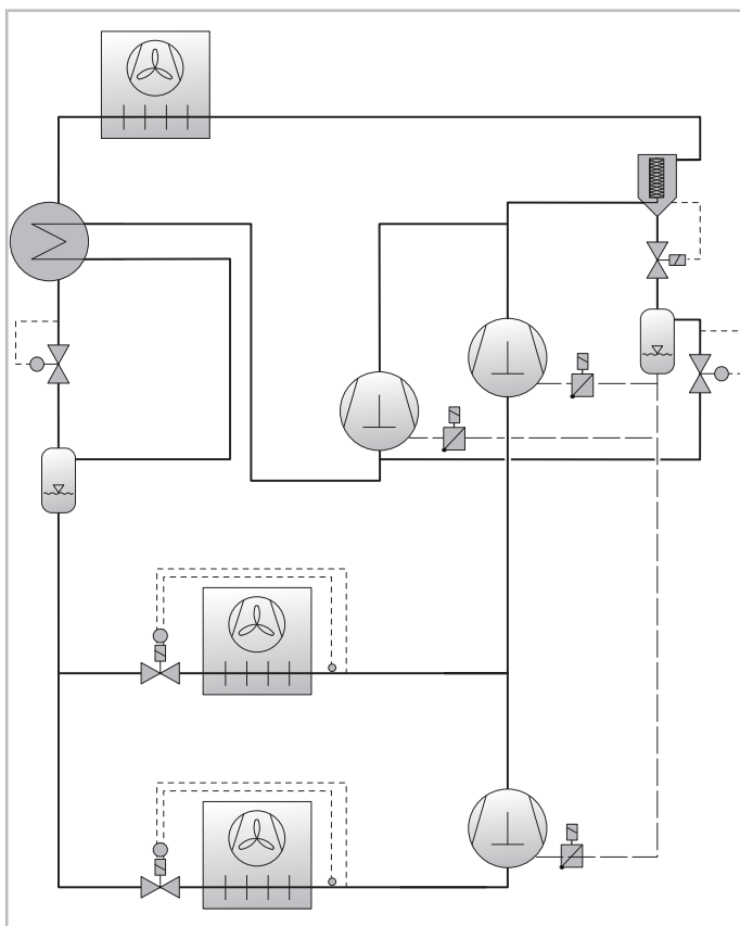
Abb. 11: Anlagenschema Booster-Anlage für Normal- und Tiefkühlung mit Parallelverdichtung (vereinfachte Darstellung)
