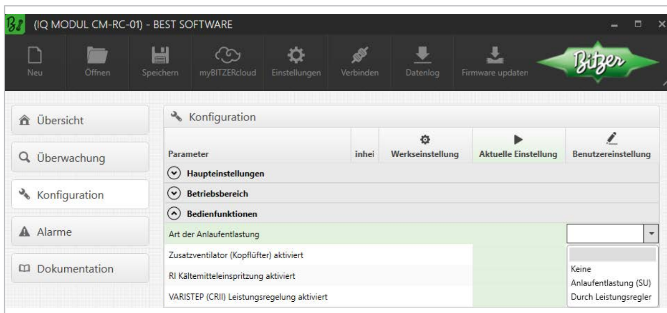
Abb. 42: Wahl der Anlaufentlastung beim CM-RC in der BEST SOFTWARE. Hat der Verdichter eine integrierte Anlaufentlastung, hier "Anlaufentlastung (SU)" wählen.
