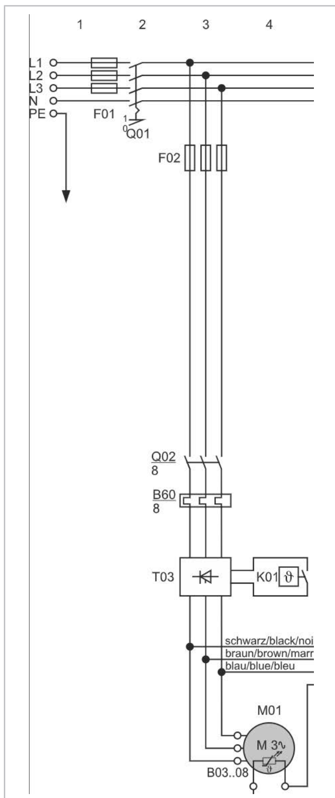
Рис. 17: Пуск с устройством плавного пуска для спирального компрессора ORBIT
