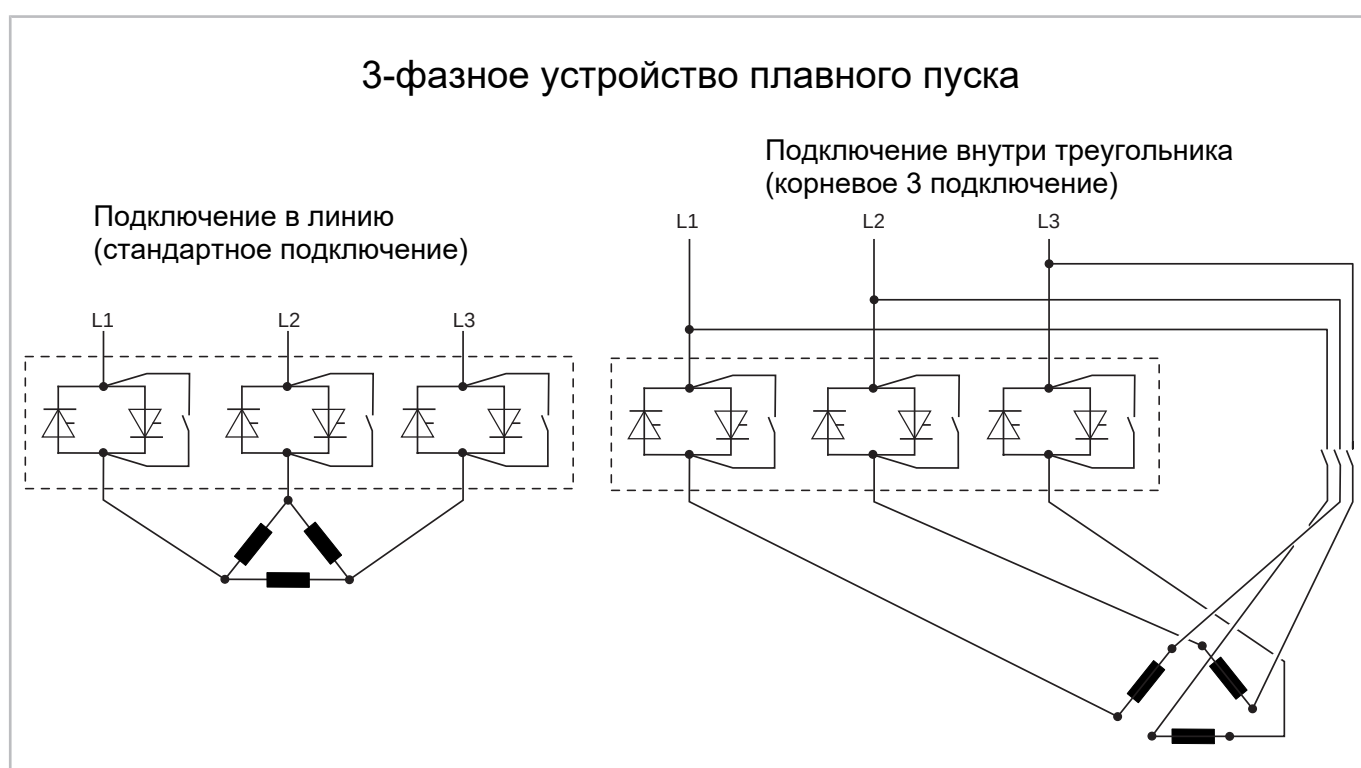
Рис. 11: Сравнение подключения между в линию и внутри треугольника для 3-фазного устройства плавного пуска
