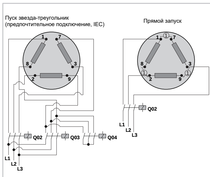
Рис. 28: Схематическое изображение внутреннего расключения мотора для пуска звезда-треугольник Q02: главный контактор (пуск звезда-треугольник) соотв. контактор компрессора (прямой пуск) Q03: контактор треугольника Q04: контактор звезды (1): перемычки для прямого пуска (опциональный аксессуар)
