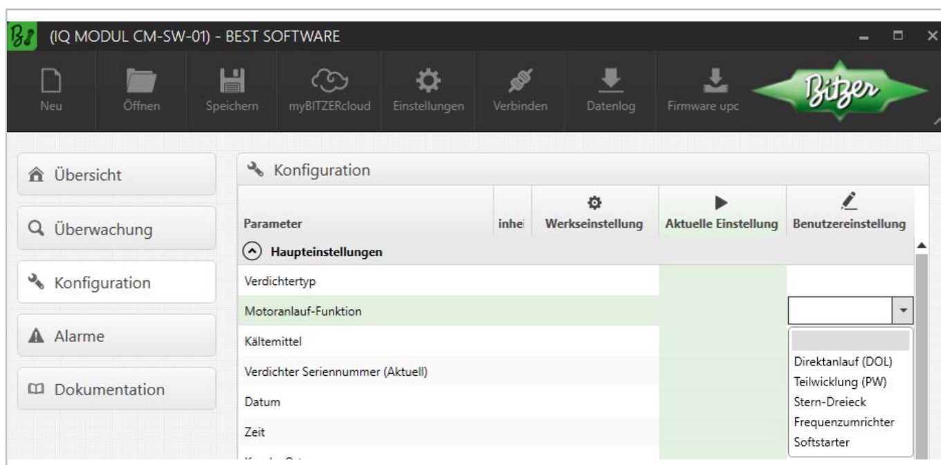
Abb. 5: Wahl des Anlaufverfahrens in der BEST SOFTWARE, hier mit CM-SW-01.
