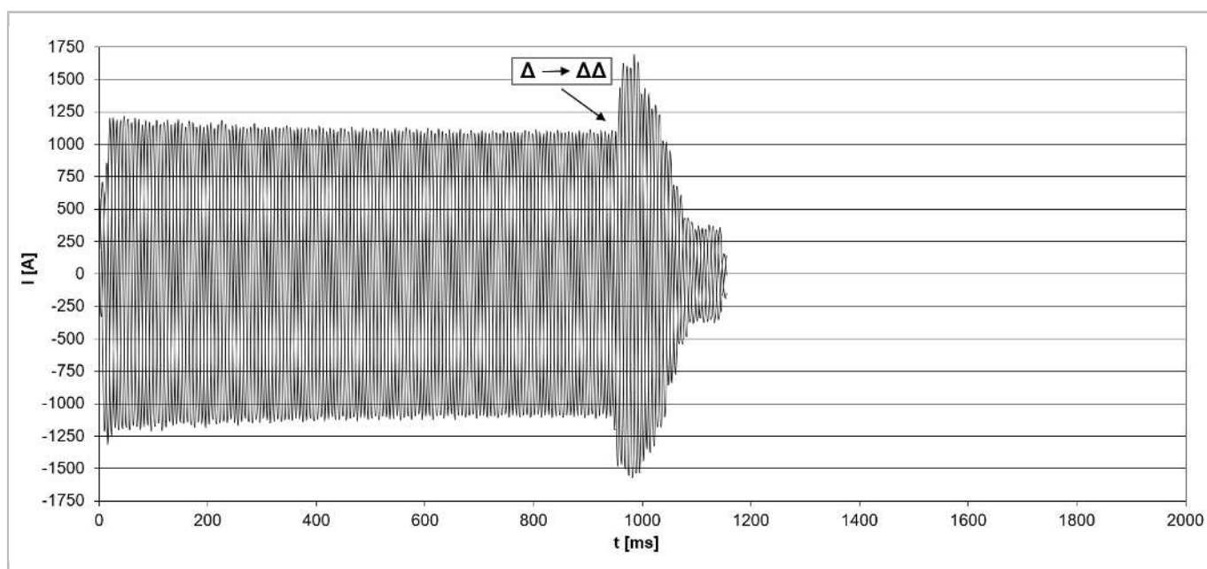
Рис. 46: Пусковой ток (пиковое значение) для компрессора модели CSH8593-180Y с пуском с разделенными обмотками (разделение 50% / 50%, тип обмотки \Delta/\Delta\Delta ) без разгрузки при пуске (например положение золотника на 100% ).
