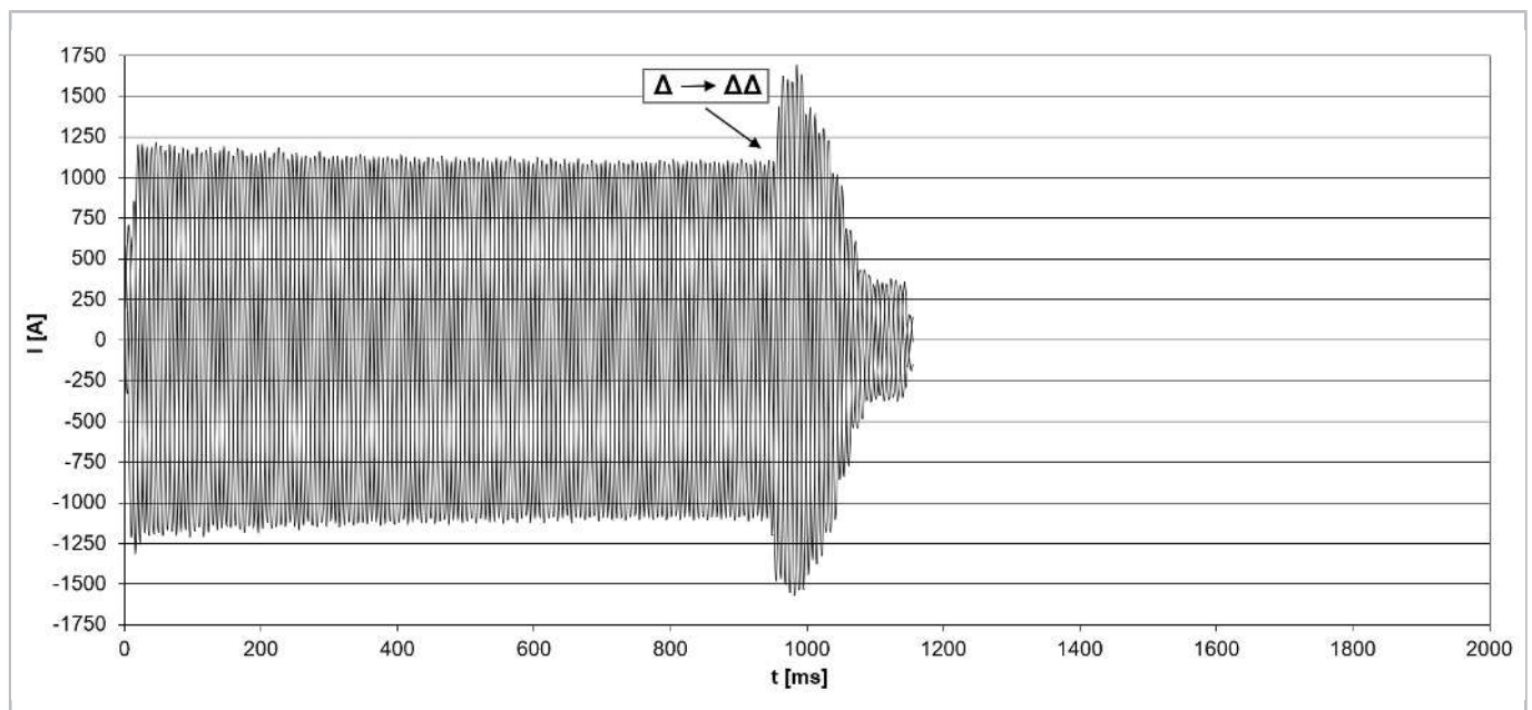
Abb. 46: Anlaufstrom (Scheitelwert) bei einem Verdichter vom Typ CSH8593-180Y mit Teilwicklungsanlauf (Wicklungsteilung 50% / 50%, Wicklungsart \Delta/\Delta\Delta ) ohne Anlaufentlastung (d.h. Schieberstellung auf 100% ).
