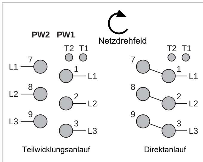
Abb. 37: Motoranschluss für Teilwicklungsanlauf HS.85 Verdichter (Beispiel)
