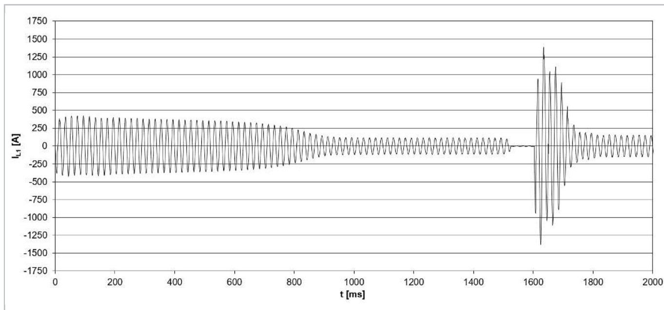
Рис. 49: Пусковой ток (пиковое значение) для компрессора модели CSH8593-140Y с пуском звезда-треугольник (IEC подключение) и пуском без нагрузки (т.е. положение золотника на 75% ).
