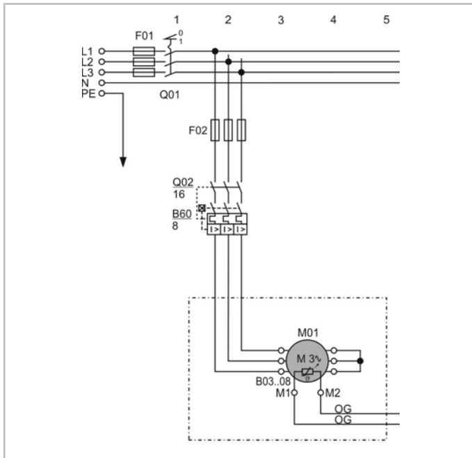
Abb. 19: Direktanlauf in Sternschaltung bei einem Hubkolbenverdichter
