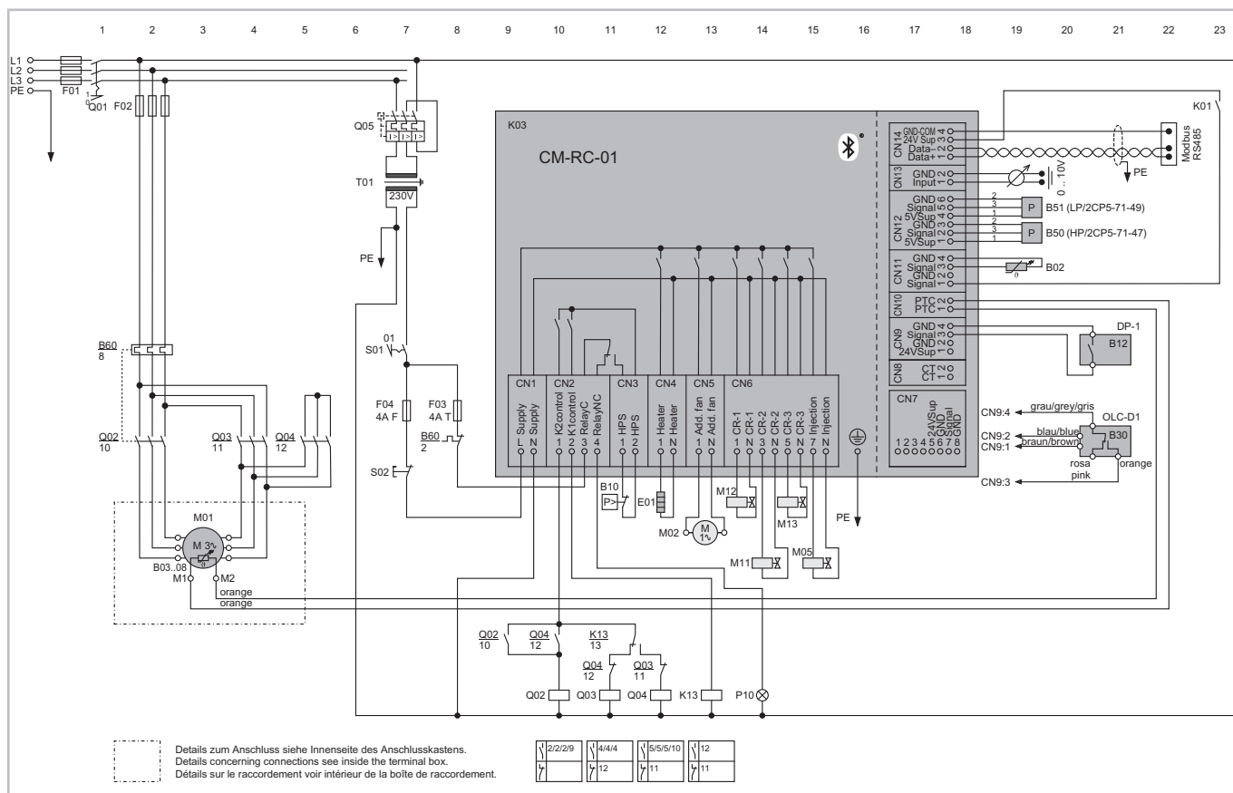
Рис. 43: Поршневой компрессор Ecoline с компрессорным модулем CM-RC-01, пуском звезда-треугольник и с разгрузкой при пуске. На схеме показано максимально возможное оснащение 6-цилиндрового компрессора с разгрузкой при пуске (электромагнитный клапан M11) и 2-мя регуляторами производительности CR11 (электромагнитные клапаны M12 и M13), размещенных здесь под компрессорным модулем CM-RC-01.
