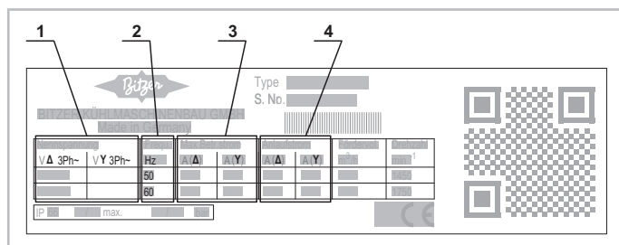
Рис. 30: Компрессор с мотором звезда-треугольник, пример заводской таблички
