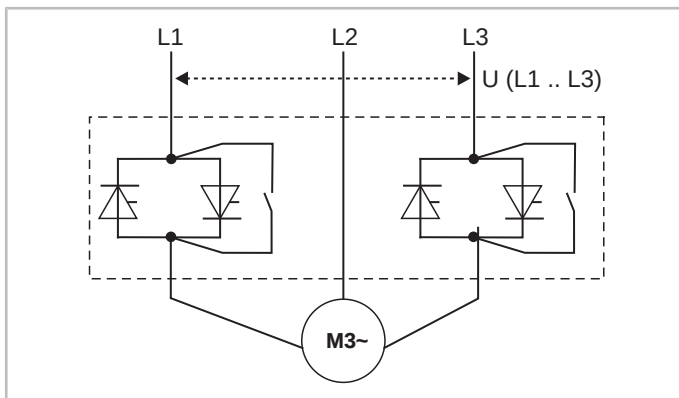
Abb. 10: Schematischer Aufbau eines 2-Phasen-gesteuerten Softstarters mit integrierten Bypasskontakten
