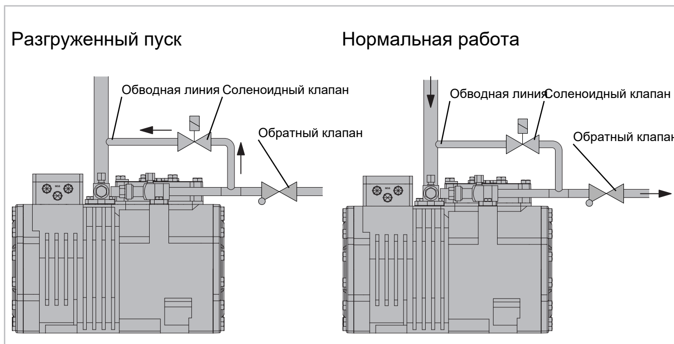
Рис. 41: Внешняя разгрузка при пуске для поршневых компрессоров BITZER (пример)
