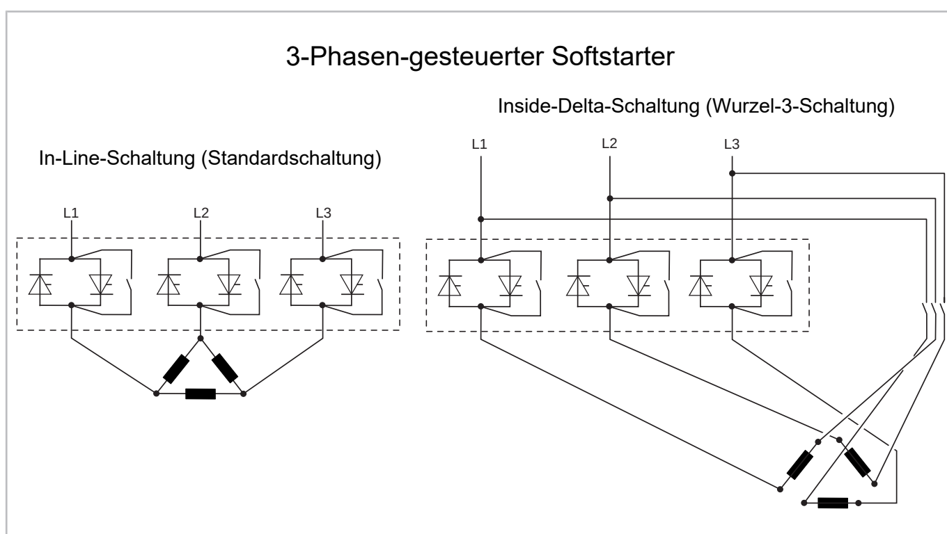
Abb. 11: Vergleich von In-Line- und Inside-Delta-Schaltung eines 3-Phasen-gesteuerten Softstarters
