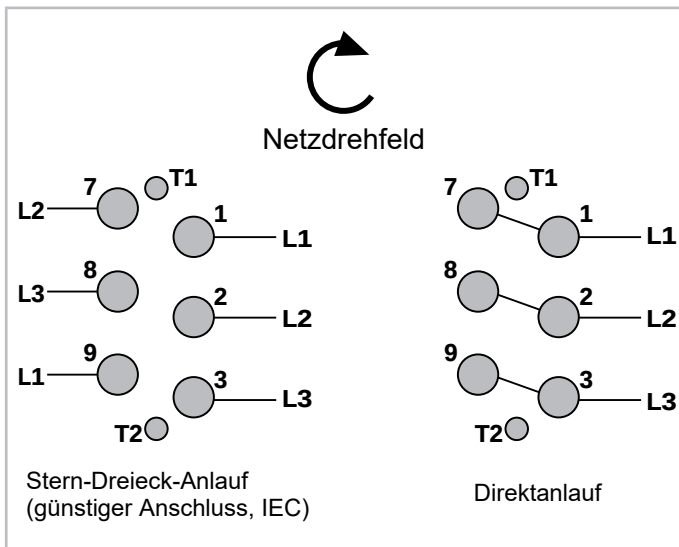
Abb. 26: Motoranschluss für Stern-Dreieck-Anlauf CS. Verdichter (Beispiel)
