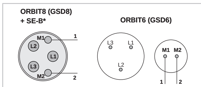
Рис. 16: Подключение мотора для пуска с помощью устройства плавного пуска для спиральных компрессоров (примеры). Для них никакое другое подключение невозможно.
