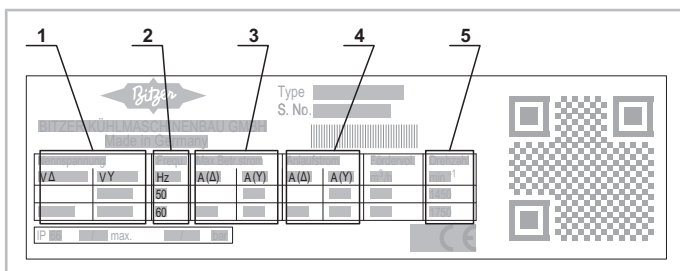
Рис. 2: Типичная заводская табличка встроенного мотора с прямым пуском, который может работать по схеме звезда или треугольник.
