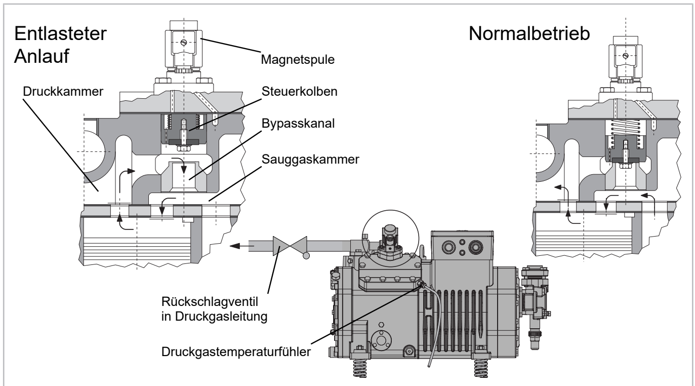
Abb. 40: Integrierte Anlaufentlastung bei BITZER Hubkolbenverdichtern (Beispiel)
