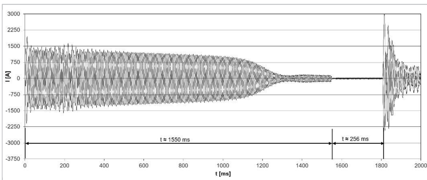
Abb. 14: Anlaufstrom (Scheitelwert) bei einem Schraubenverdichter vom Typ CSW10593-360Y mit Stern-Dreieck-Anlauf. Der Anlaufstrom (Rotor blockiert) beträgt 955 A (Stern) / 2913 A (Dreieck).
