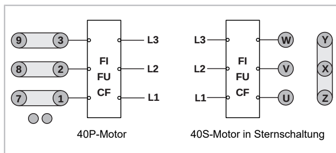
Abb. 6: Motoranschlüsse an der Stromdurchführungsplatte bei Betrieb mit externem Frequenzumrichter (FU), Beispiele für Hubkolbenverdichter
