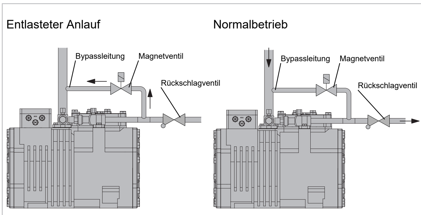
Abb. 41: Externe Anlaufentlastung bei BITZER Hubkolbenverdichtern (Beispiel)
