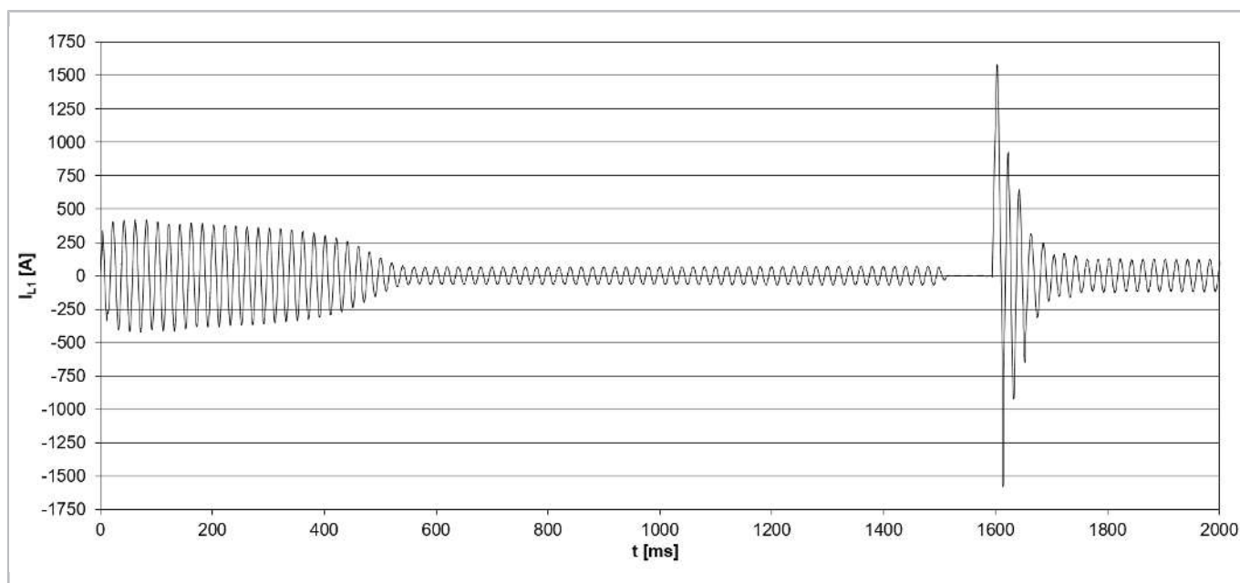
Рис. 48: Пусковой ток (пиковое значение) для компрессора модели CSH8593-140Y с пуском звезда-треугольник (IEC подключение) и пуском без нагрузки (т.е. положение золотника на 50% ).
