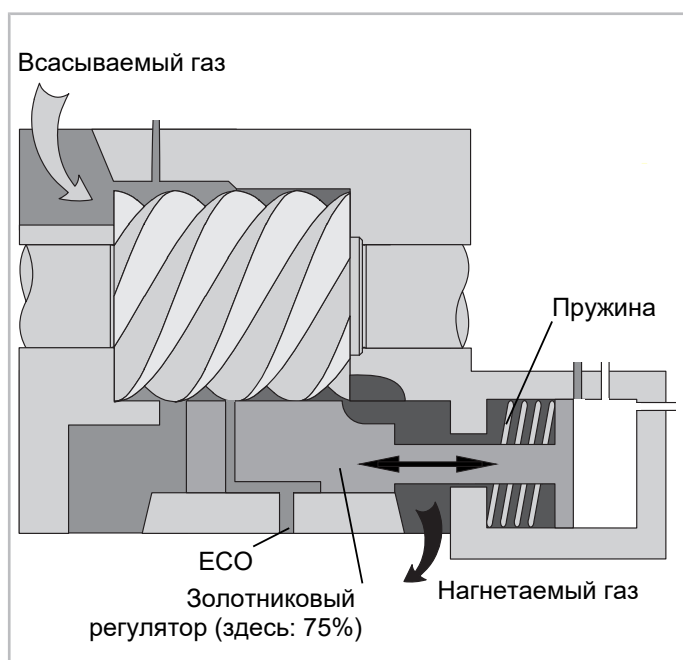
Рис. 44: Принцип золотникового регулирования, например для CS. винтовых компрессоров BITZER
