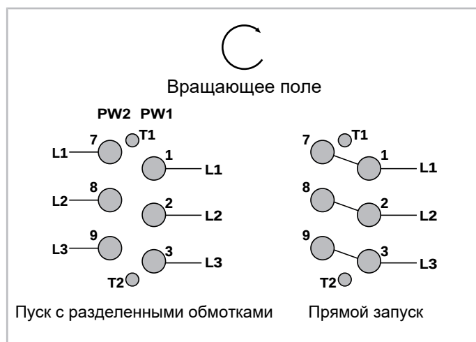
Рис. 36: Подключение мотора для пуска с разделенными обмотками для CS.85 компрессора (пример)
