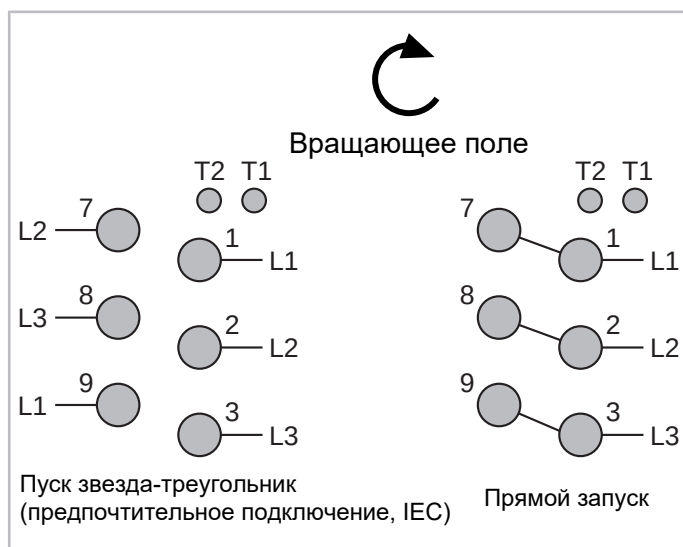
Рис. 27: Подключение мотора для компрессора HS.85 с пуском звезда-треугольник (пример)
