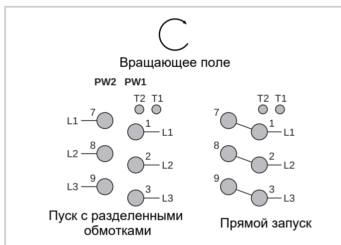
Рис. 37: Подключение мотора для пуска с разделенными обмотками для HS.85 компрессора (пример)
