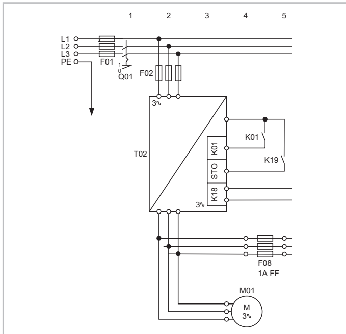
Abb. 8: Anlauf mit Frequenzumrichter bei einem OS.95 Schraubenverdichter
