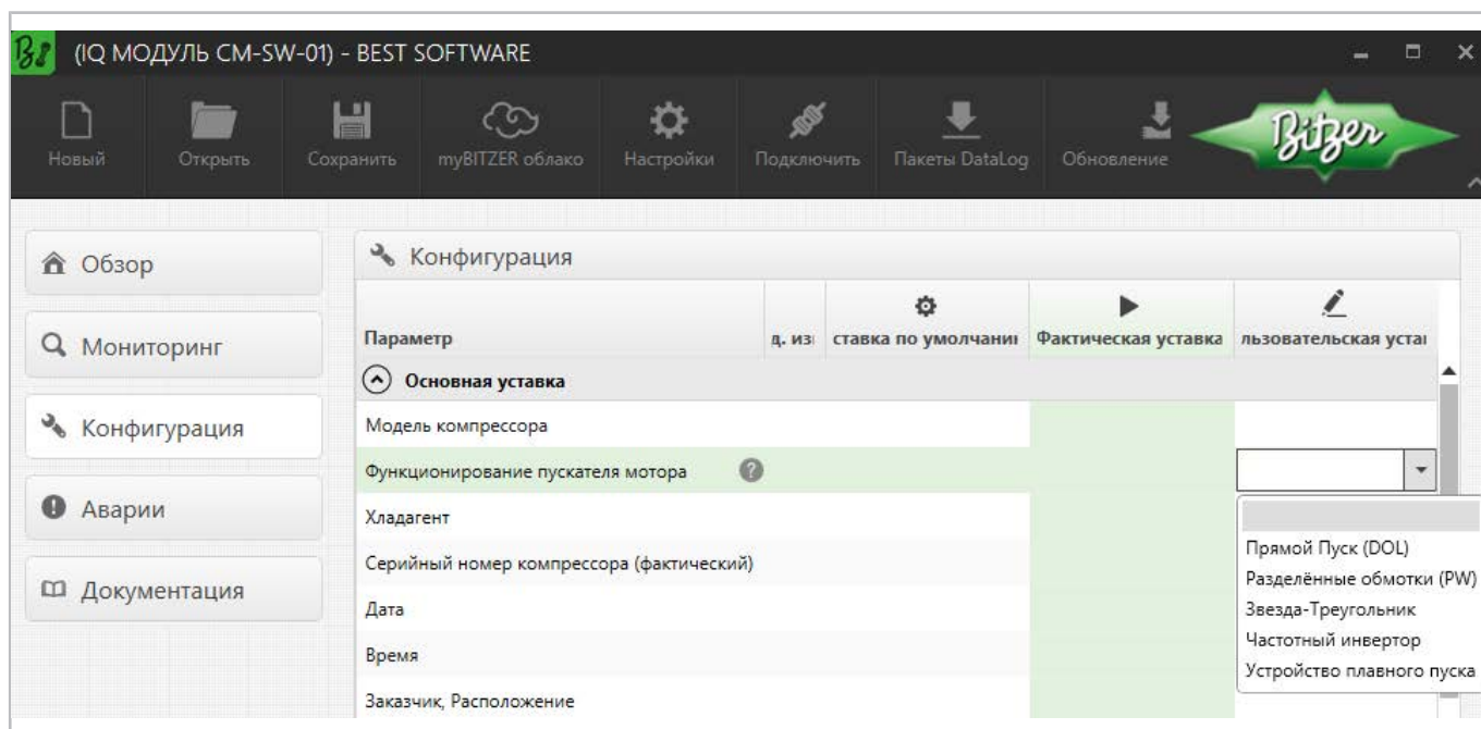
Рис. 5: Выбор метода пуска в BEST SOFTWARE, в данном случае с CM-SW-01.
