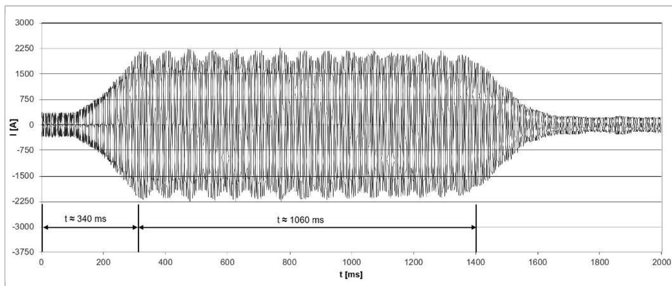
Рис. 13: Пусковой ток (пиковое значение) винтового компрессора модели CSW10593-360Y с устройством плавного пуска. Его макс. рабочий ток 565 A.
