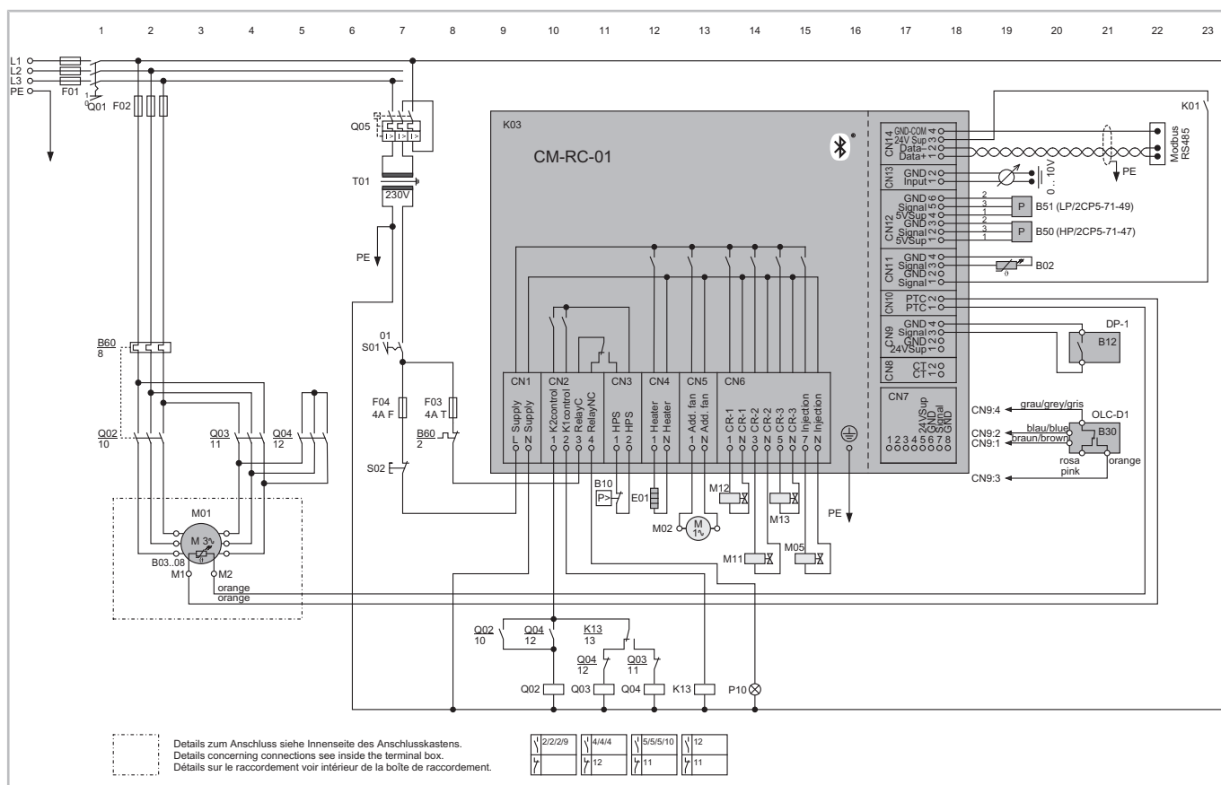
Abb. 43: ECOLINE Hubkolbenverdichter mit Verdichtermodul CM-RC-01, Stern-Dreieck-Anlauf und Anlaufentlastung. Gezeigt ist eine theoretische Maximalausstattung eines 6-Zylinder-Verdichters mit Anlaufentlastung (Magnetventil M11) und 2-mal CRII Leistungsregelung (Magnetventile M12 und M13), hier zu sehen unter dem Verdichtermodul CM-RC-01.
