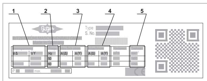
Abb. 2: Typisches Typschild für einen eingebauten Direktanlaufmotor, der im Stern oder im Dreieck betrieben werden kann.
