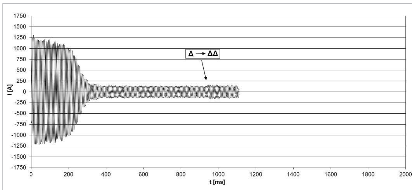
Рис. 45: Пусковой ток (пиковое значение) для компрессора модели CSH8593-180Y с разделенными обмотками (разделение 50%/50%, тип обмотки \Delta/\Delta\Delta ) и с разгруженным пуском (т.е. положение золотника на 25% ).
