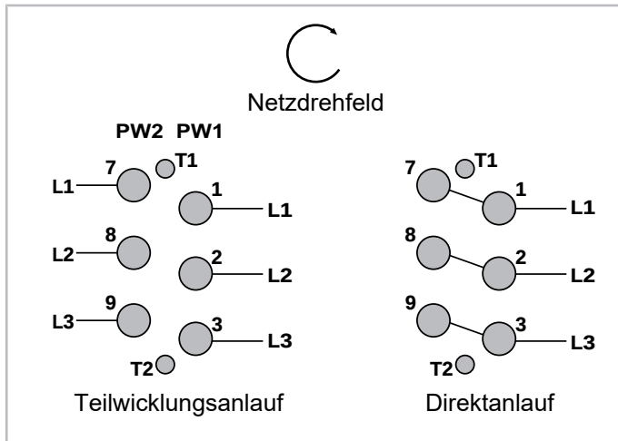
Abb. 36: Motoranschluss für Teilwicklungsanlauf CS.85 Verdichter (Beispiel)
