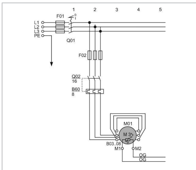
Рис. 20: Прямой пуск по схеме треугольник для поршневого компрессора
