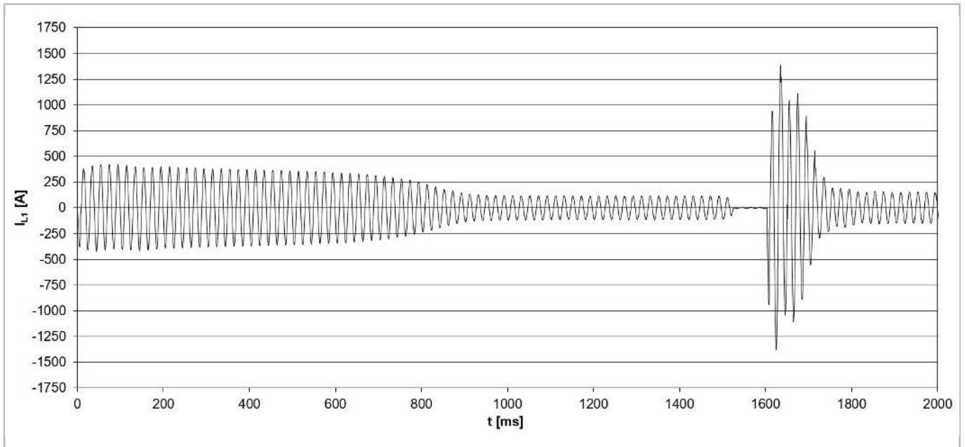
Abb. 49: Anlaufstrom (Scheitelwert) bei einem Verdichter vom Typ CSH8593-140Y mit Stern-Dreieck-Anlauf (IEC-Schaltung) und Anlaufentlastung (durch Schieberstellung auf 75% ).
