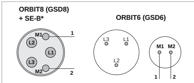
Abb. 16: Motoranschluss für Anlauf mit Softstarter bei BITZER Scrollverdichtern (Beispiele). Bei diesen sind keine anderen Anschlüsse möglich.
