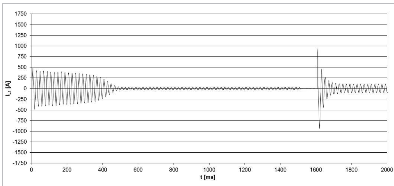
Рис. 47: Пусковой ток (пиковое значение) для компрессора модели CSH8593-140Y с пуском звезда-треугольник (IEC подключение) и пуском без нагрузки (т.е. положение золотника на 25% ).
