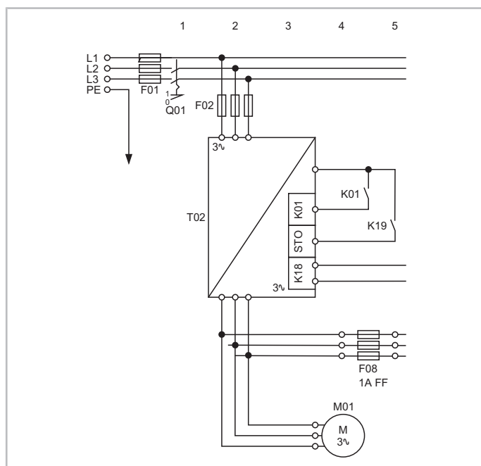
Рис. 8: Пуск с преобразователем частоты винтового компрессора OS.95
