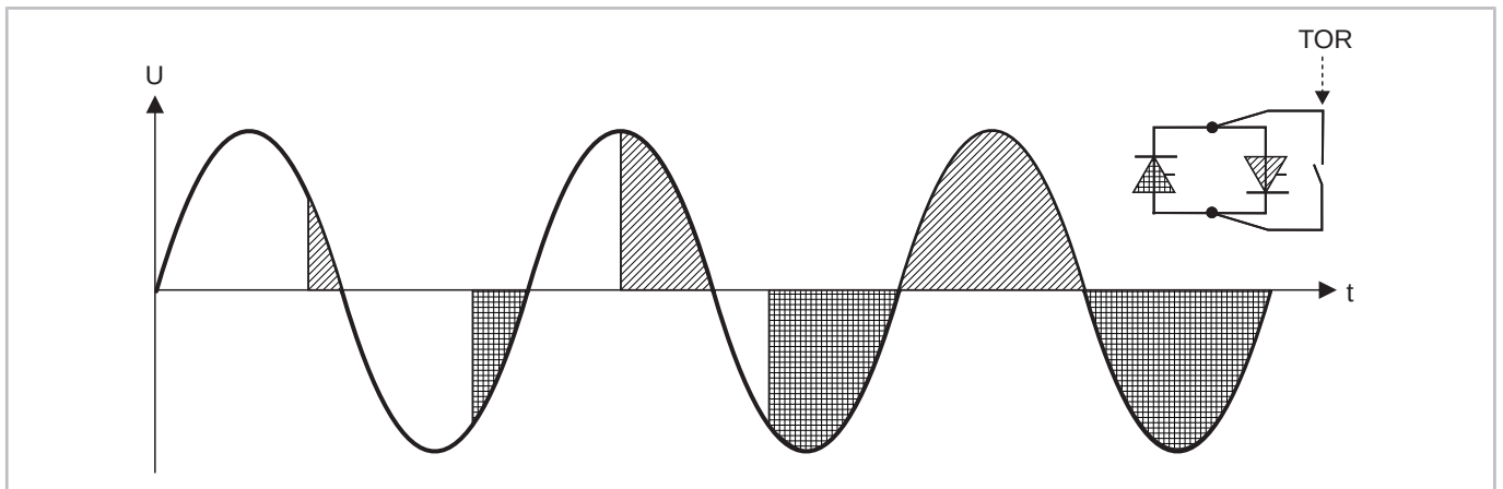
Abb. 9: Softstarter: Phasenanschnittsteuerung und Bypass-Kontakt (TOR: "top of ramp", volle Sinushalbwellen).
