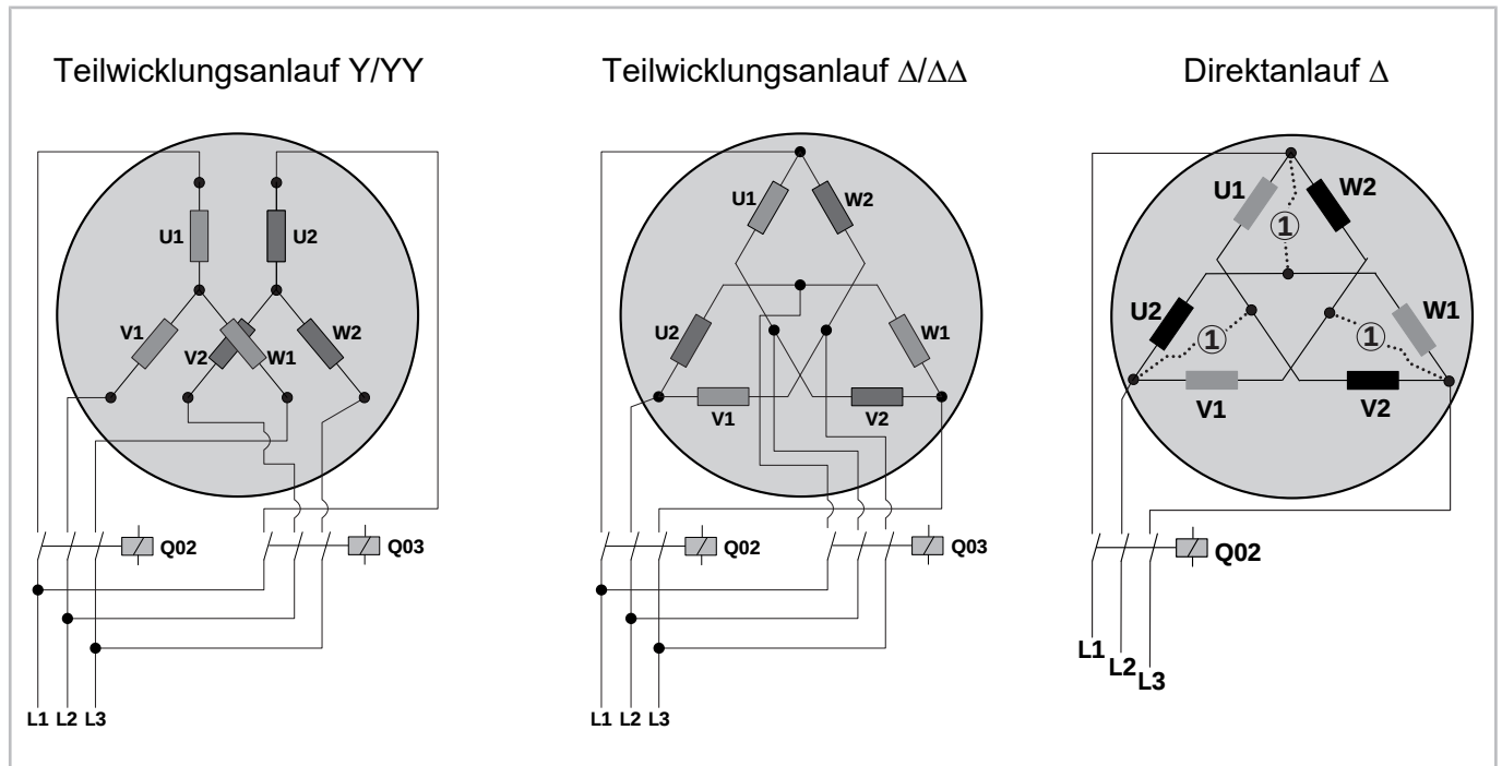
Abb. 38: Schematische Darstellung der internen Schaltung im Motor bei Teilwicklungsanlauf
