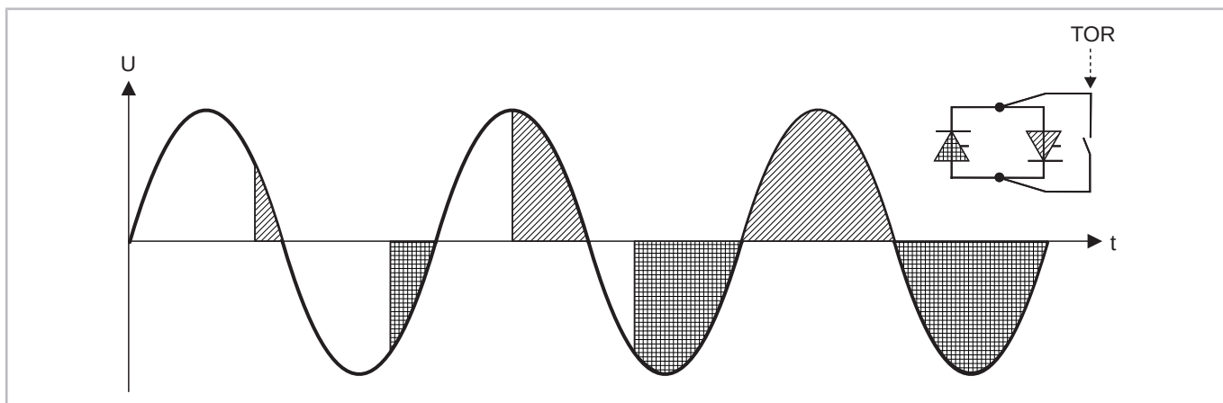
Рис. 9: Устройство плавного пуска: контроль фазового угла и обходной контакт (TOR: вершина рампы, полные синусоидальные полу-волны).
