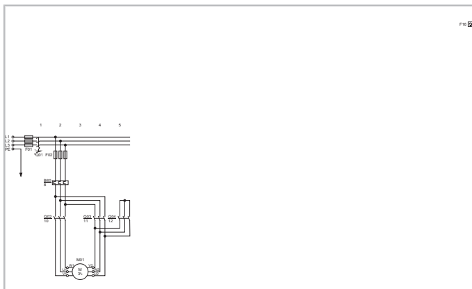
Abb. 29: Stern-Dreieck-Anlauf bei einem OS.85 Schraubenverdichter
