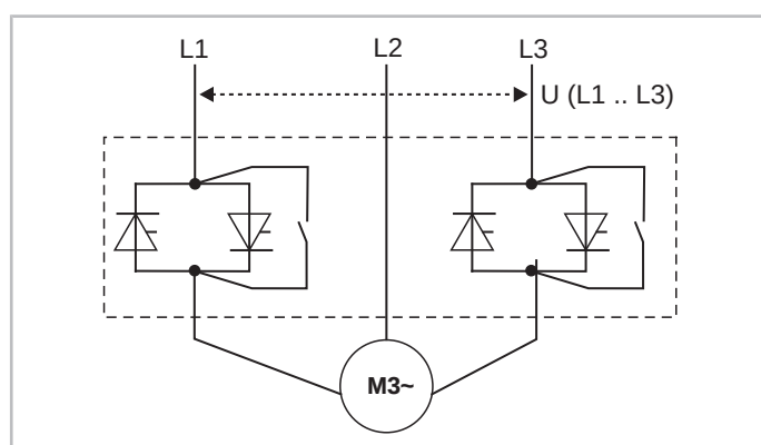
Рис. 10: Схематическая структура 2-фазного устройства плавного пуска со встроенными контактами байпаса
