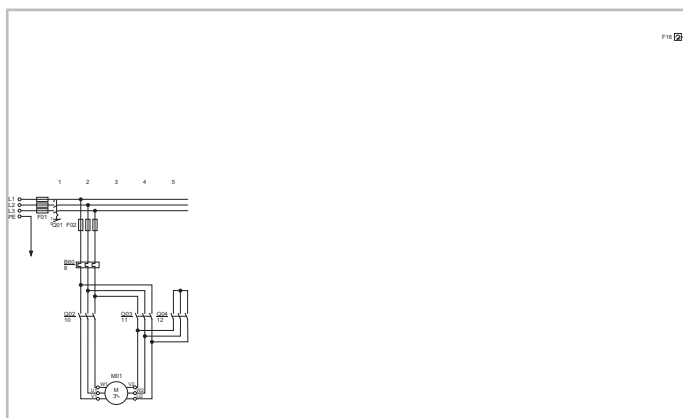
Рис. 29: Пуск звезда-треугольник для винтового компрессора OS.85 Q02: главный контактор Q03: контактор треугольника Q04: контактор звезды M01: мотор
