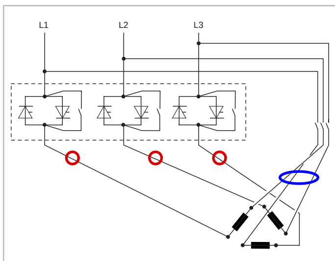
Рис. 12: Рекомендуемое подключение контроля направления вращения к 3-фазному устройству плавного пуска с подключением внутри треугольника: либо в точках красных кругов, либо в точках синего эллипса.
