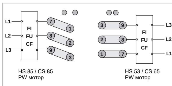
Рис. 7: Клеммы мотора на клеммной колодке для работы с внешним преобразователем частоты (FI), примеры для винтовых компрессоров
