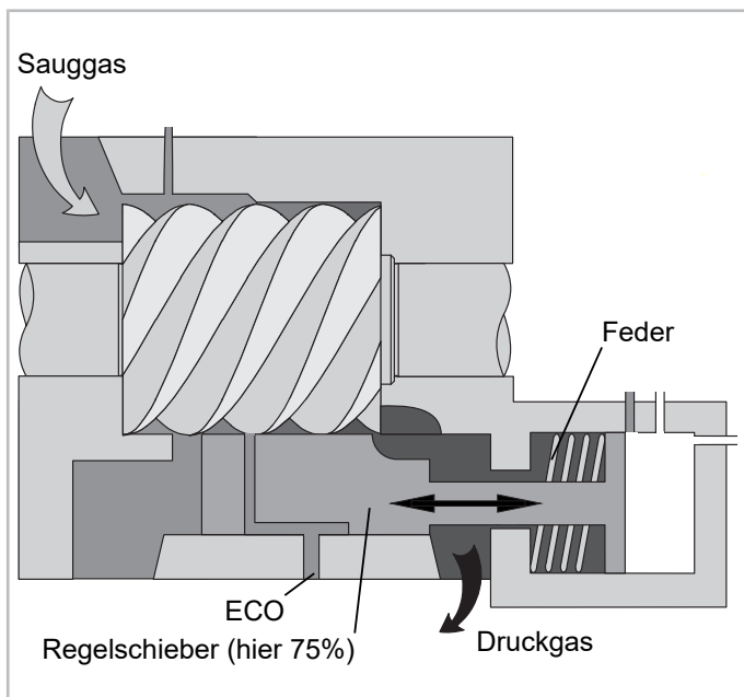
Abb. 44: Prinzip der Schiebersteuerung z.B. bei einem BITZER CS. Schraubenverdichter
