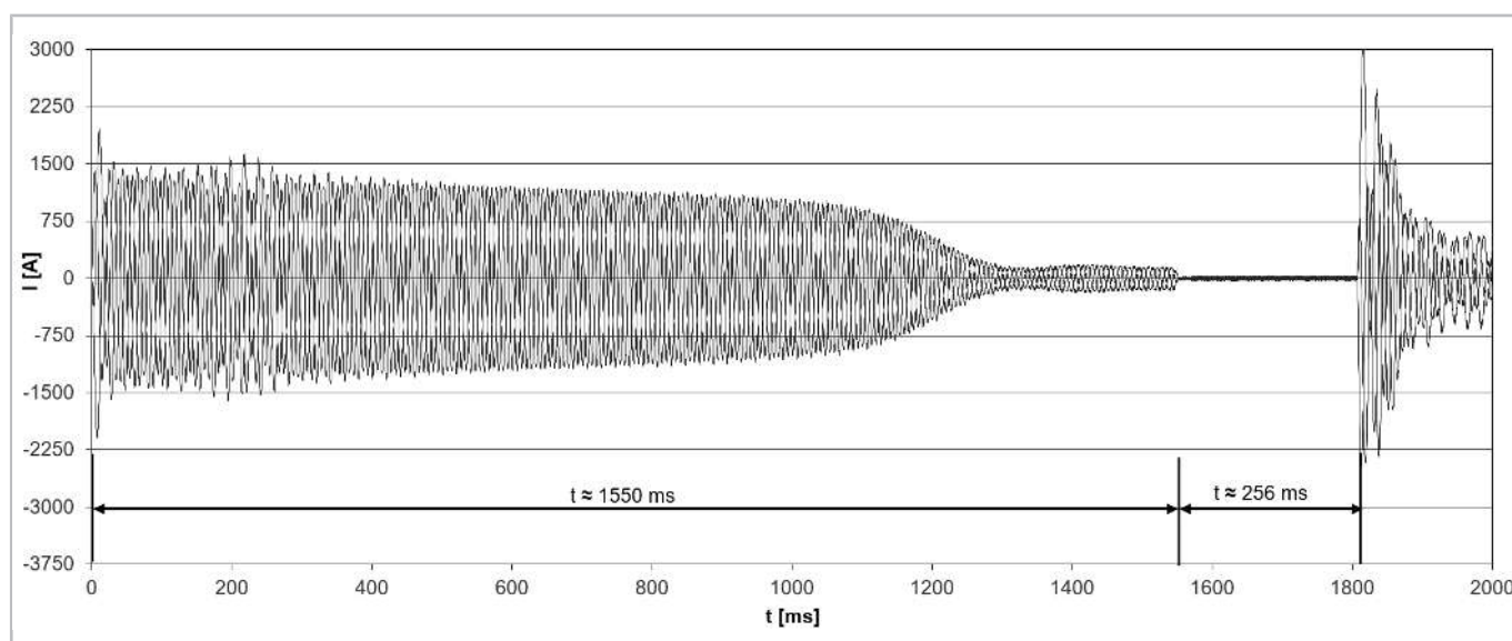
Рис. 14: Пусковой ток (пиковое значение) винтового компрессора модели CSW10593-360Y с подключением звезда-треугольник. Пусковой ток (ротор заблокирован) составляет 955 A (звезда) / 2913 A (треугольник).
