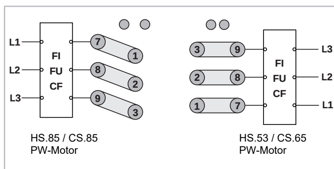
Abb. 7: Motoranschlüsse an der Stromdurchführungsplatte bei Betrieb mit externem Frequenzumrichter (FU), Beispiele für Schraubenverdichter
