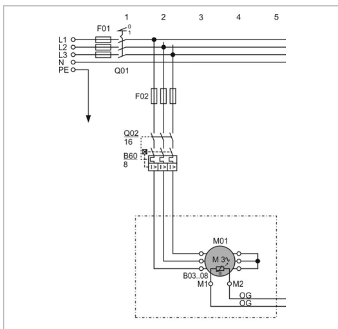
Рис. 19: Прямой пуск по схеме звезда для поршневого компрессора
