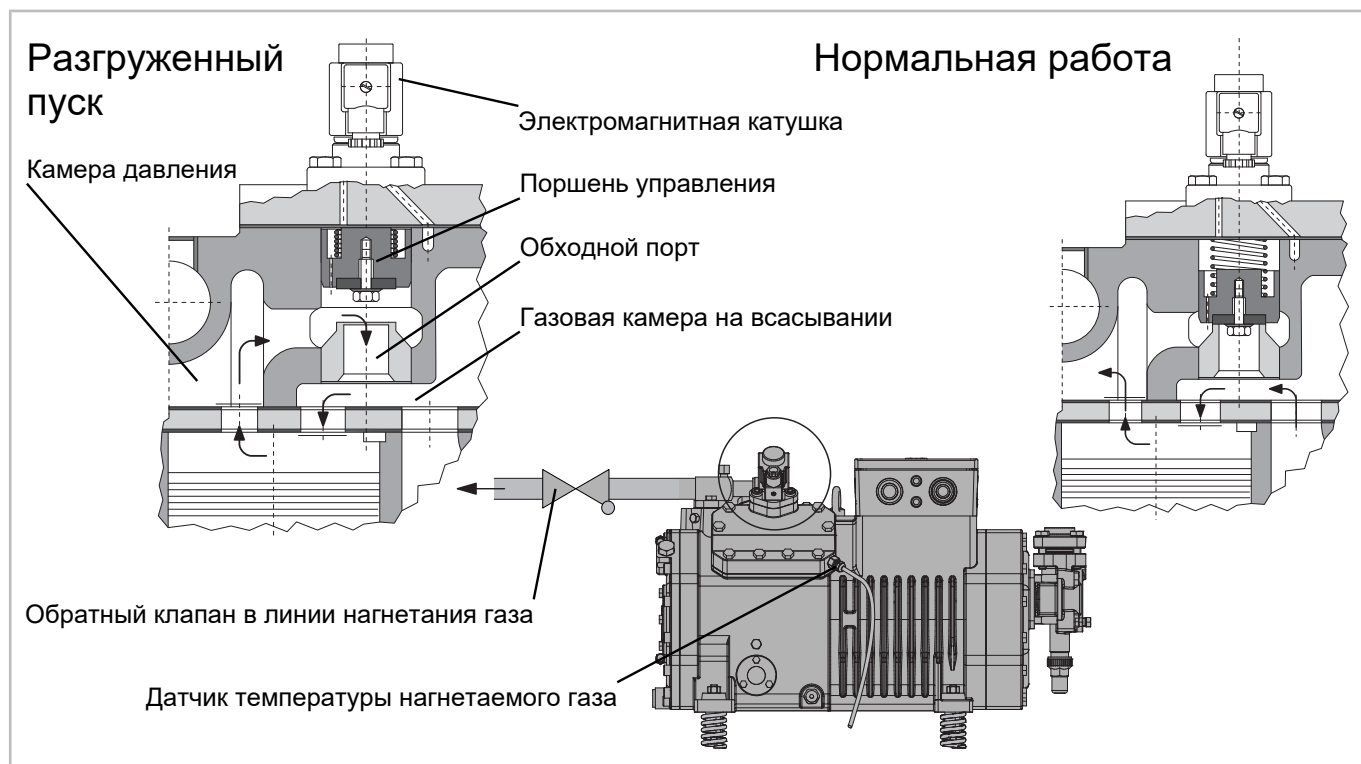
Рис. 40: Интегрированная разгрузка при пуске для поршневых компрессоров BITZER (пример)
