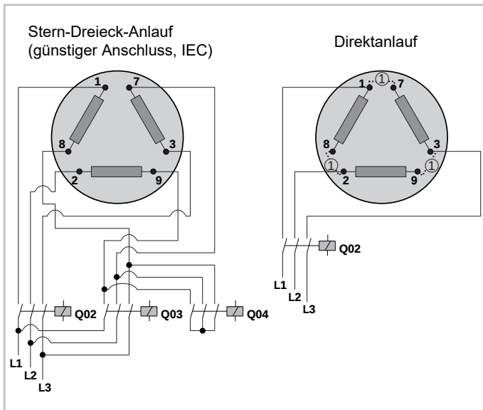
Abb. 28: Schematische Darstellung der internen Schaltung im Motor bei Stern-Dreieck-Anlauf
