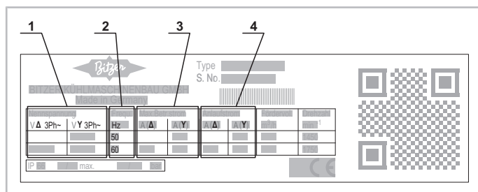
Abb. 21: Verdichter mit Direktanlaufmotor, Beispiel eines Typschilds
