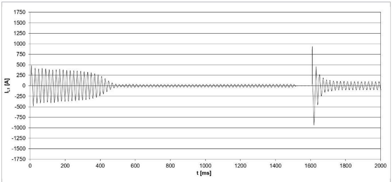
Abb. 47: Anlaufstrom (Scheitelwert) bei einem Verdichter vom Typ CSH8593-140Y mit Stern-Dreieck-Anlauf (IEC-Schaltung) und Anlaufentlastung (durch Schieberstellung auf 25% ).
