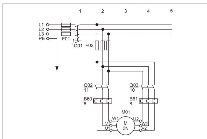
Рис. 39: Пуск с разделенными бмотками для винтового компрессора OS.85
