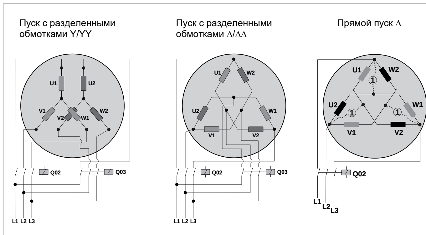
Рис. 38: Схематическое изображение внутреннего расключения мотора для пуска с разделенной обмоткой
