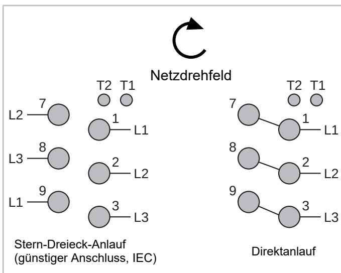
Abb. 27: Motoranschluss für Stern-Dreieck-Anlauf HS.85 Verdichter (Beispiel)
