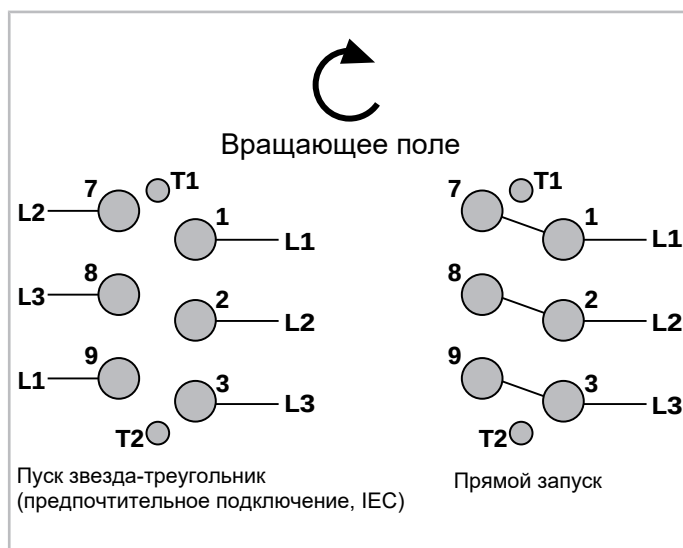
Рис. 26: Подключение мотора CS. для пуска звезда-треугольник компрессор (пример)
