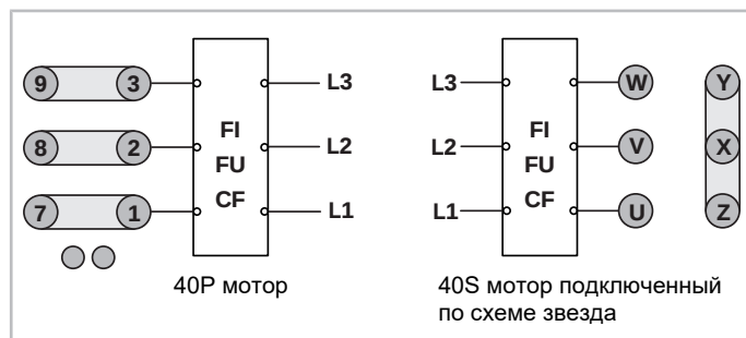
Рис. 6: Клеммы мотора на клеммной колодке для работы с внешним преобразователем частоты (FI), примеры для поршневых компрессоров
