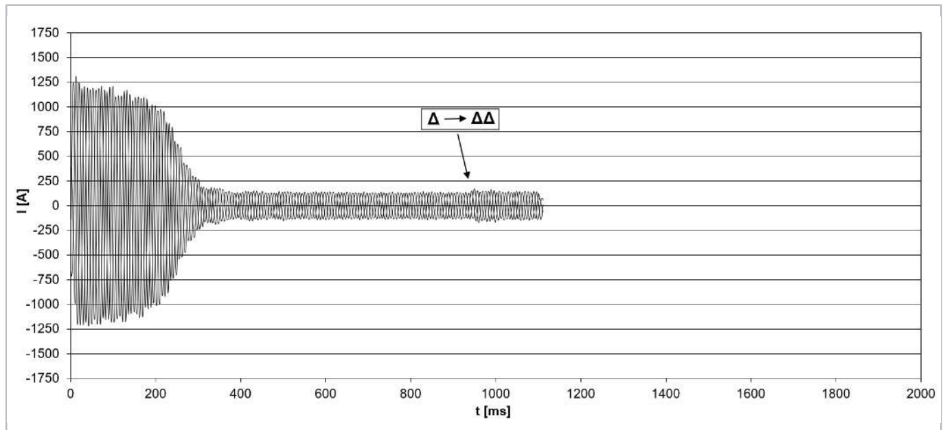
Abb. 45: Anlaufstrom (Scheitelwert) bei einem Verdichter vom Typ CSH8593-180Y mit Teilwicklungsanlauf (Wicklungsteilung 50% / 50%, Wicklungsart \Delta/\Delta\Delta ) und Anlaufentlastung (durch Schieberstellung auf 25% ).
