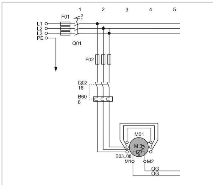
Abb. 20: Direktanlauf in Dreieckschaltung bei einem Hubkolbenverdichter
