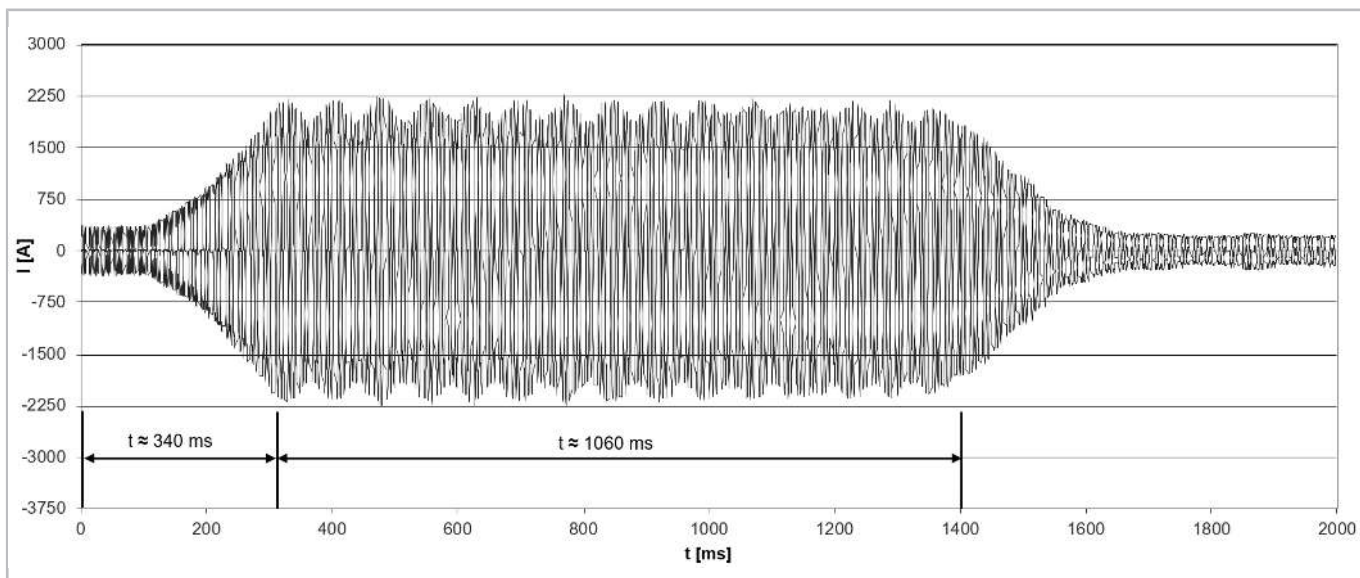
Abb. 13: Anlaufstrom (Scheitelwert) bei einem Schraubenverdichter vom Typ CSW10593-360Y mit Softstarter. Sein max. Betriebsstrom beträgt 565 A.
