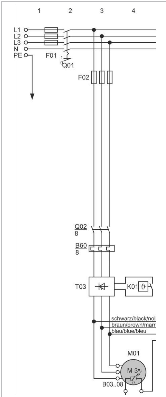
Abb. 17: Anlauf mit Softstarter bei einem ORBIT Scrollverdichter
