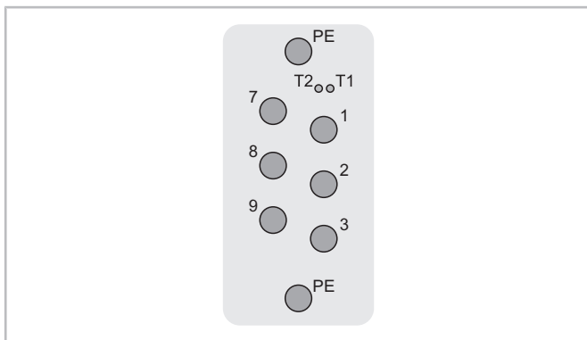
Abb. 22: Stromdurchführungsplatte
