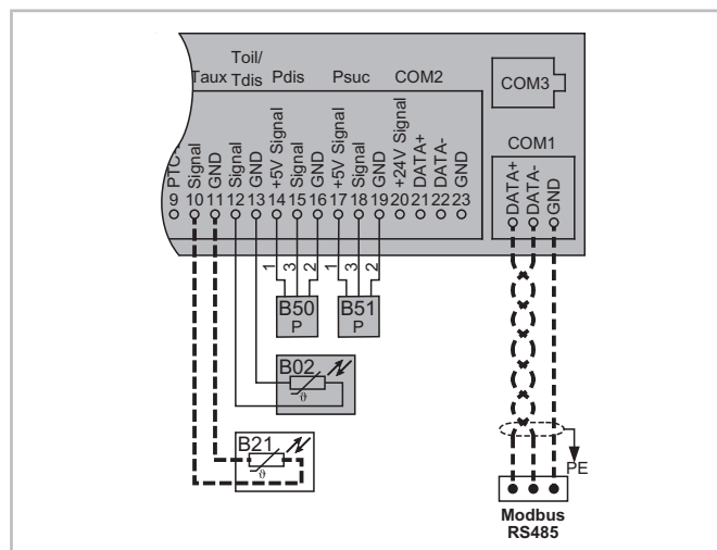
Fig. 36: SE-i1 à HS., partie 2 : Les trois sondes: transmetteur de haute et de et basse pression (B50, B51) et la sonde de température de gaz de refoulement (B02) sont montés sur le compresseur à l'état de livraison et raccordés électriquement. Modbus et une sonde de température optionnelle (B21) peuvent être raccordés. Pour les deux sondes de température (B02 et B21), il faut utiliser des sondes CTN.
