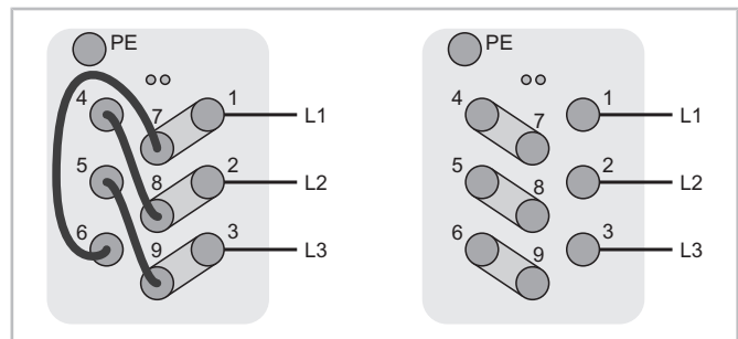
Fig. 20: Raccordement pour démarrage direct, à gauche pour la basse tension indiquée sur la plaque signalétique, à droite pour la haute tension.
