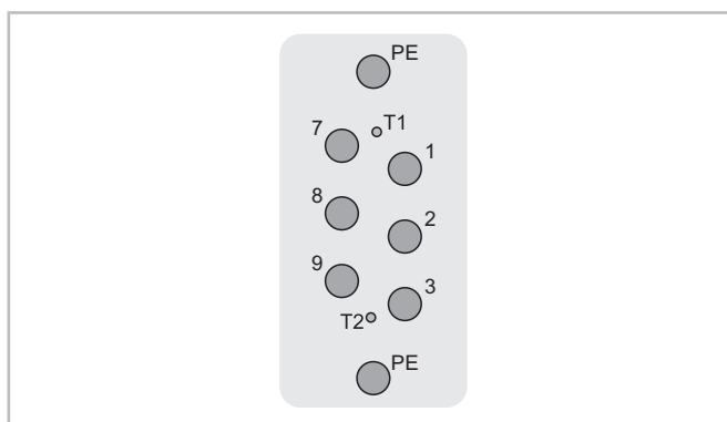
Abb. 21: Stromdurchführungsplatte
