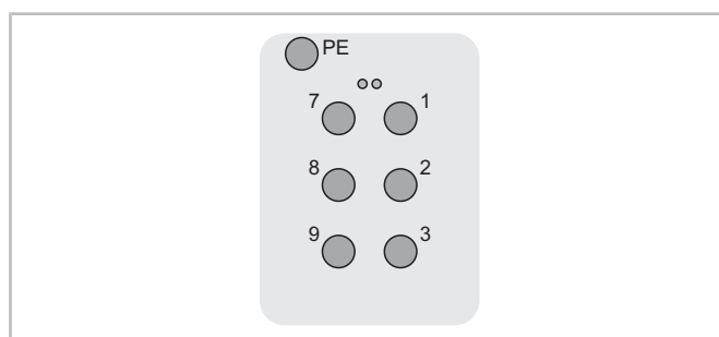
Abb. 18: Stromdurchführungsplatte
