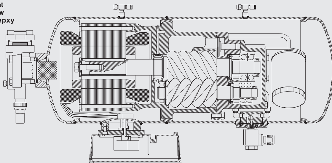
Abb. 1 Schnitt VSK41
