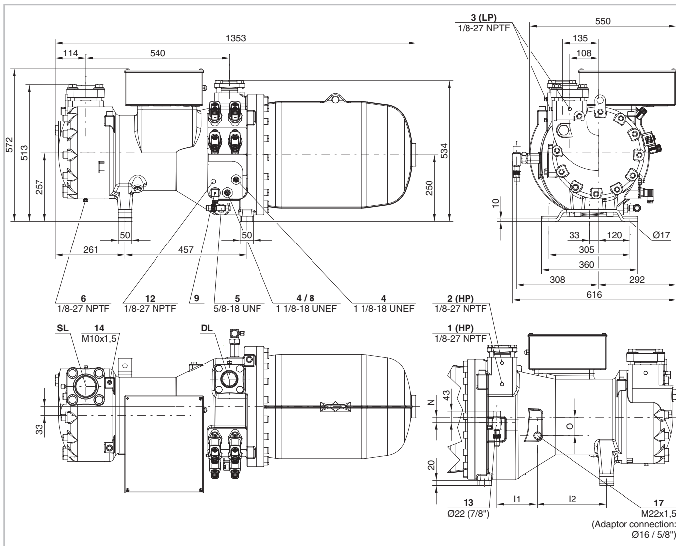
Abb. 13: Maßzeichnung CSW7573-60Y .. CSW7593-90(Y), CSH7673-70Y .. CSH7693-90Y
