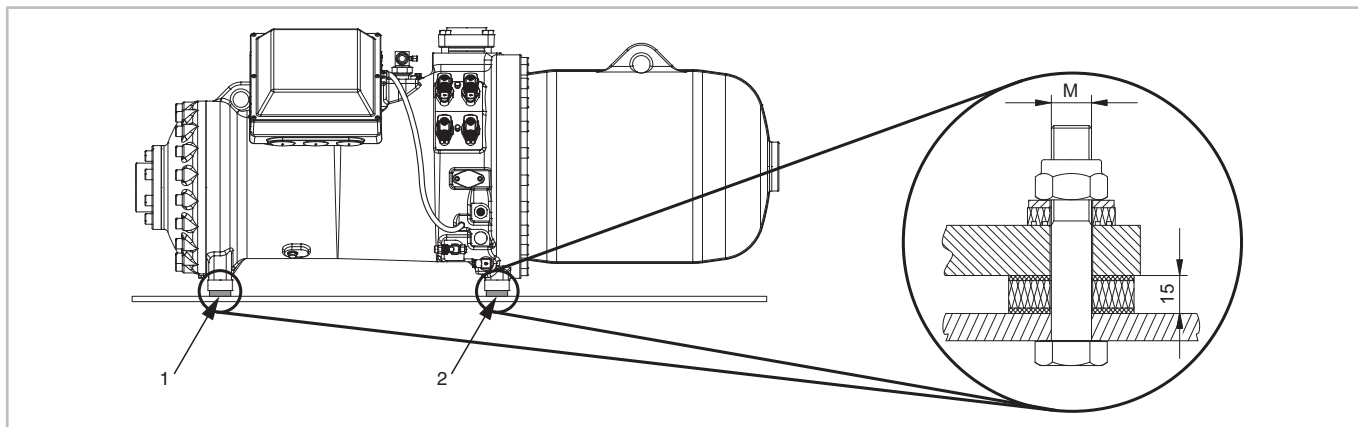
Abb. 4: Schwingungsdämpfer
