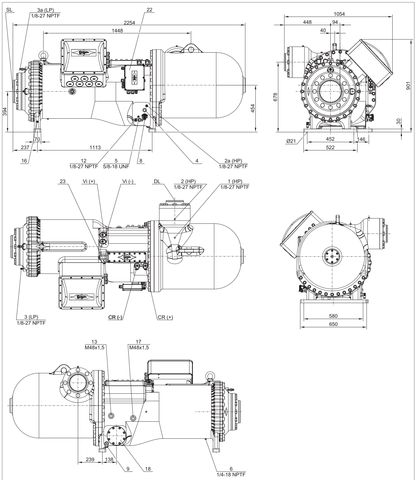
Abb. 16: Maßzeichnung CSW10593-400Y
