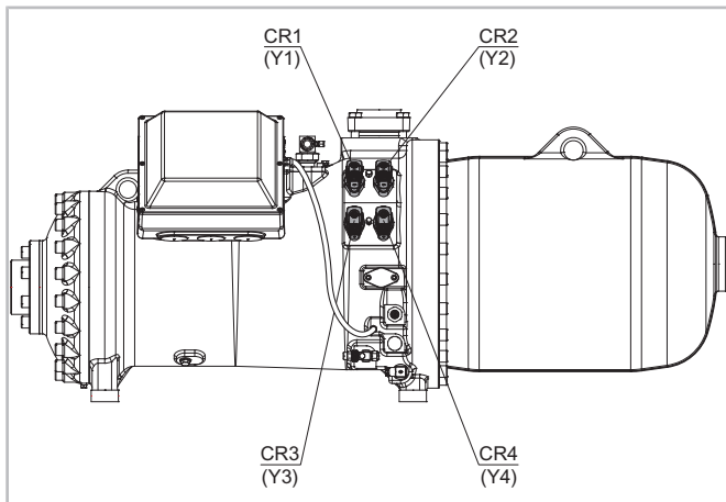
Abb. 7: Anordnung Magnetventile
