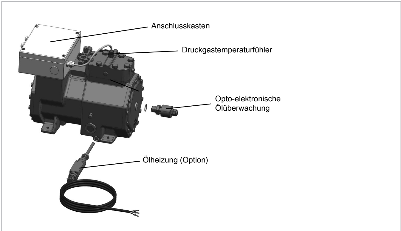
Abb. 3: 2KES(P)-05.EX(Y/P) .. 2FES(P)-3.EX(Y/P)
