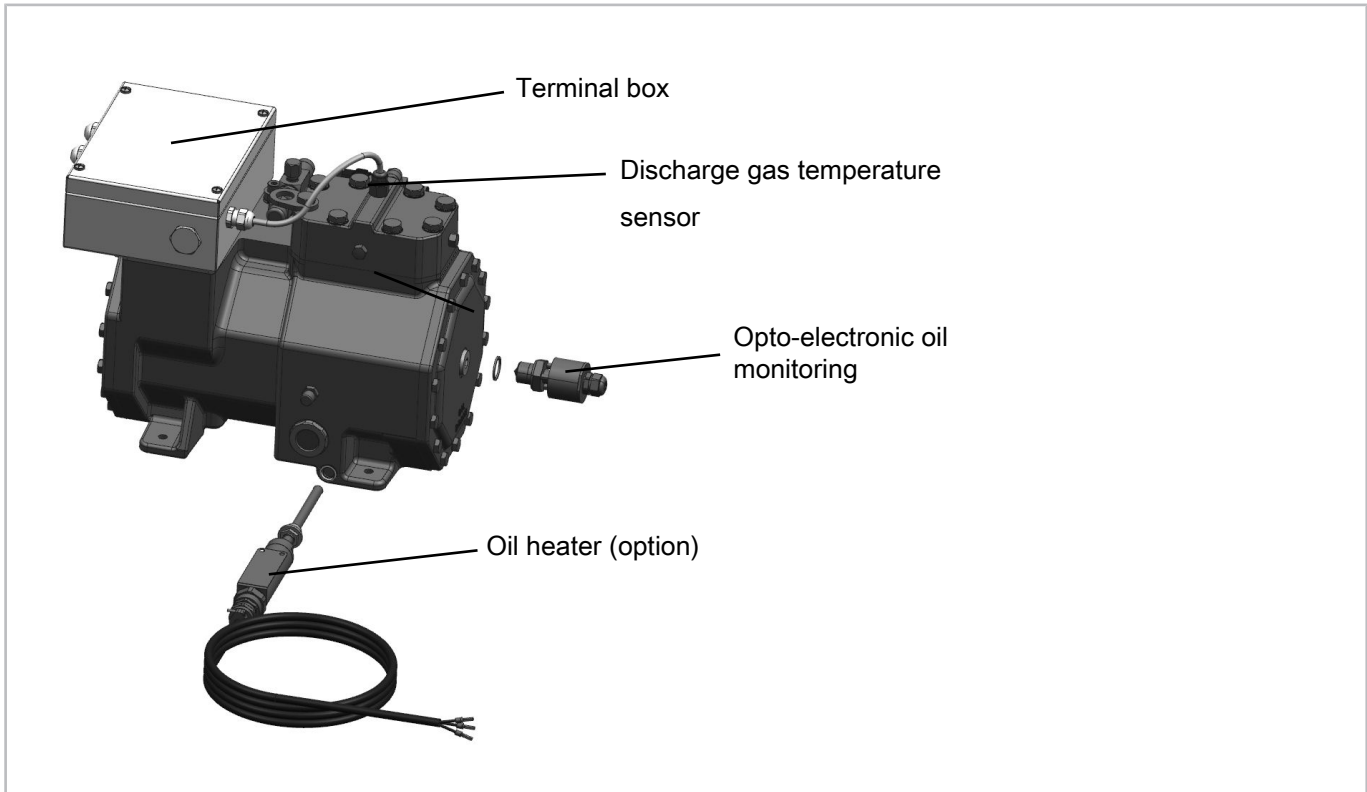
Fig. 3: 2KES(P)-05.EX(Y/P) .. 2FES(P)-3.EX(Y/P)
