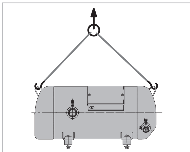
Fig. 3: Soulever le compresseur
