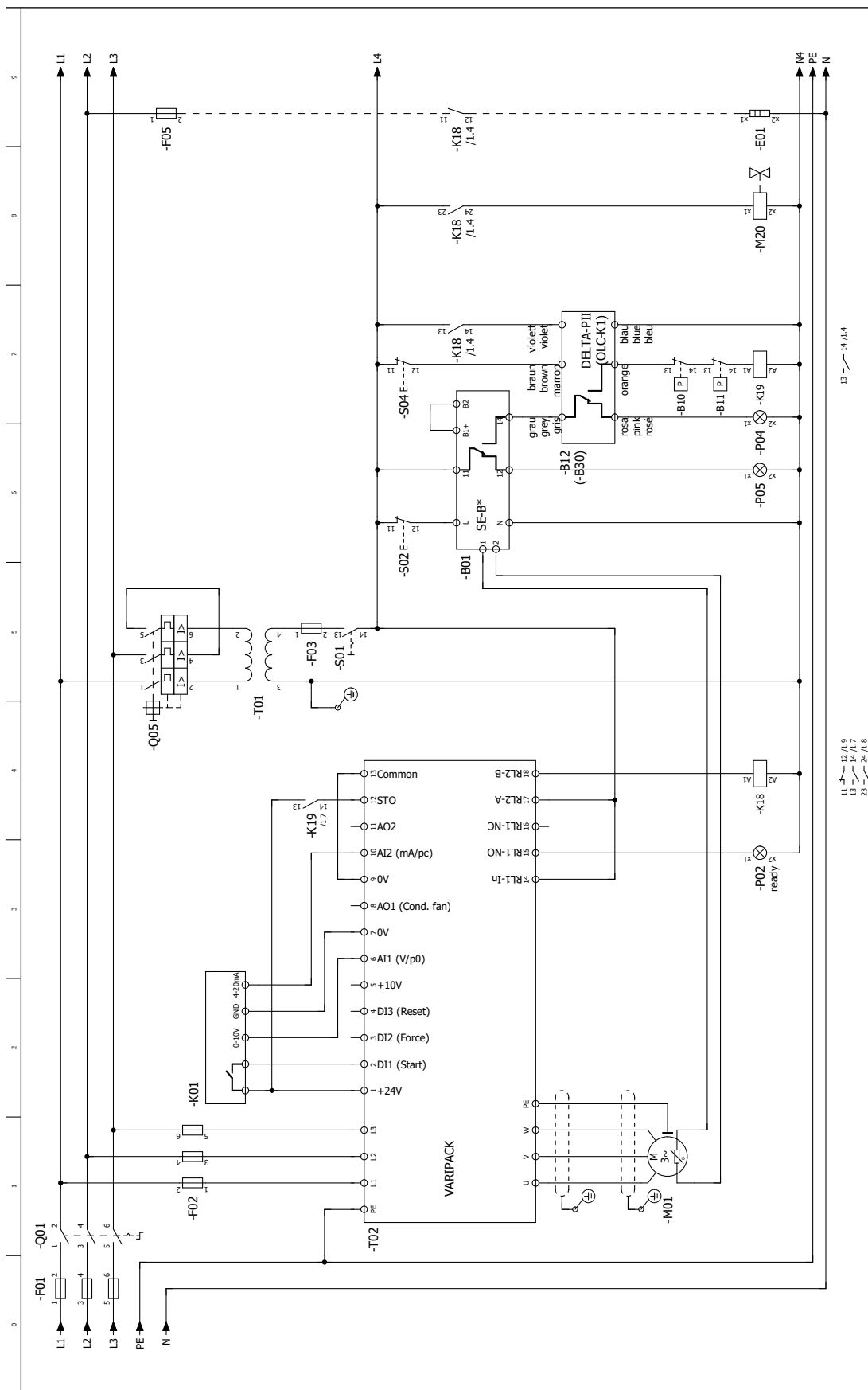
Abb. 12: Schaltbild Hubkolbenverdichter ohne Erweiterungsmodul
