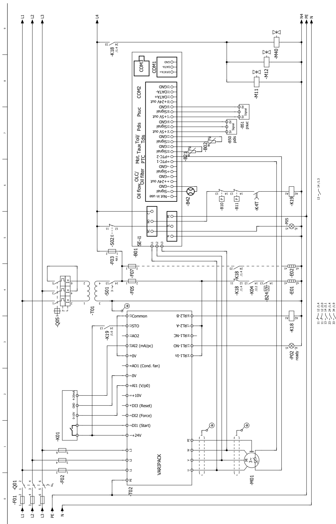
Abb. 14: HS.53 .. HS.74-Schraubenverdichter ohne Erweiterungsmodul
