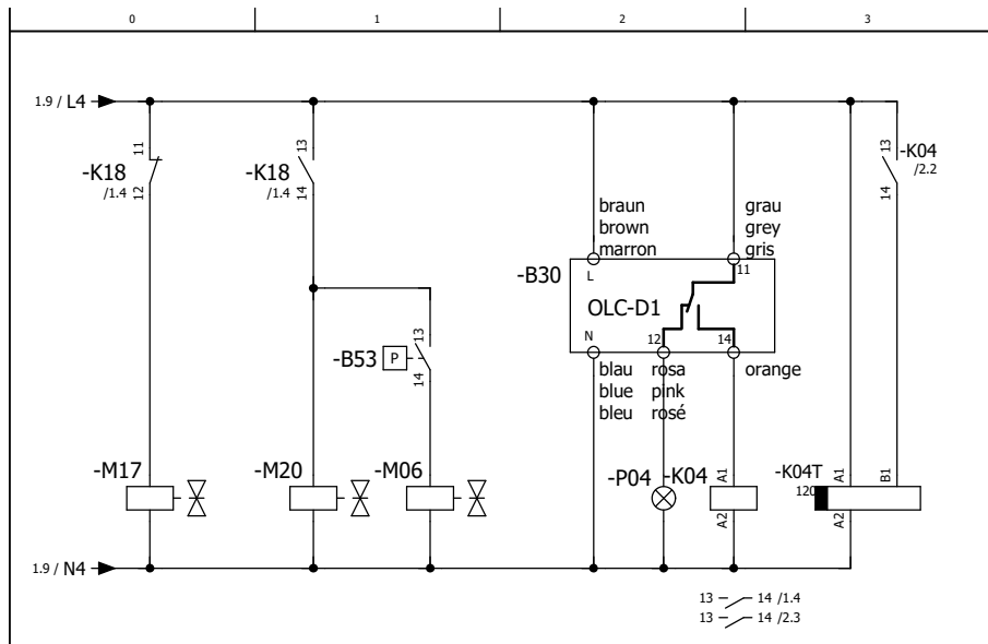
Fig. 17: Contrôle d'huile pour compresseurs à vis HS.85
