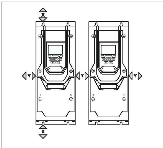
Abb. 3: Mindestbelüftungsabstände
